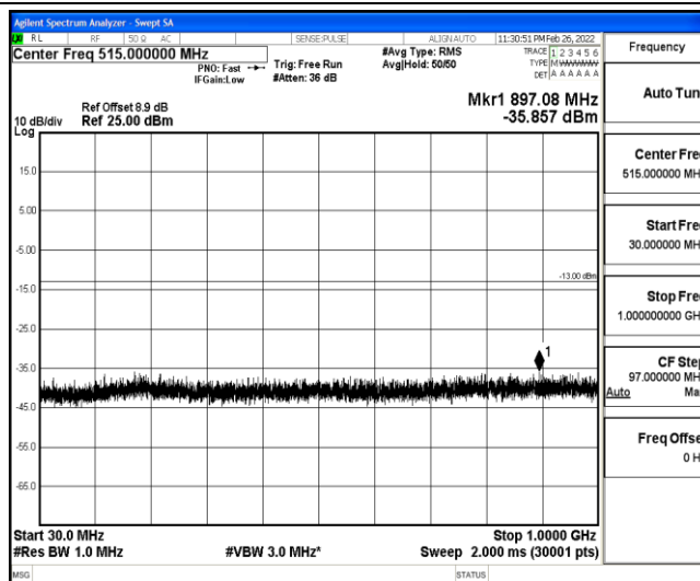
Band25-10MHz-16QAM-26365-1-0-Low-30-1000--35.86-PASS
