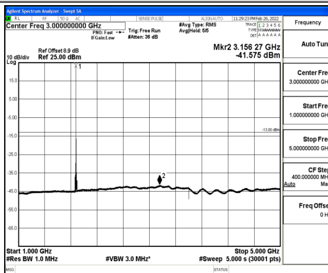
Band25-10MHz-QPSK-26365-1-0-Low-1000-5000--41.58-PASS
