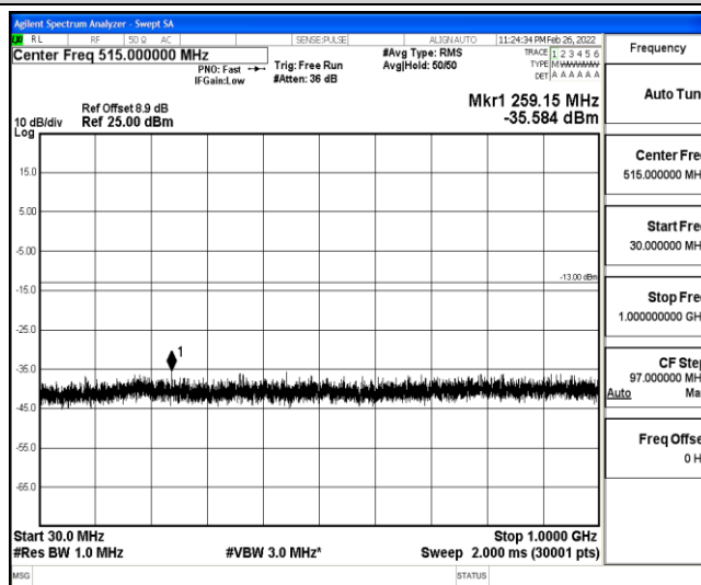
Band25-10MHz-QPSK-26090-1-0-Low-30-1000--35.58-PASS
