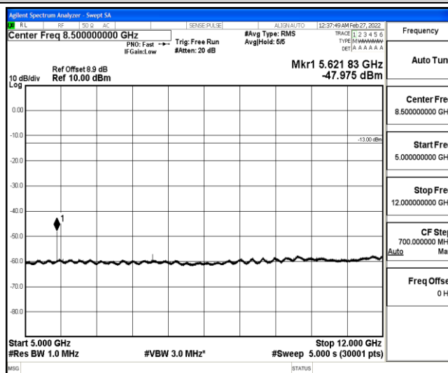
Band25-20MHz-QPSK-26365-1-0-Low-5000-12000--47.98-PASS
