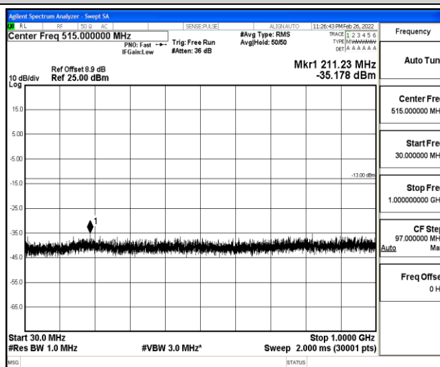
Band25-10MHz-16QAM-26090-1-0-Low-30-1000--35.18-PASS
