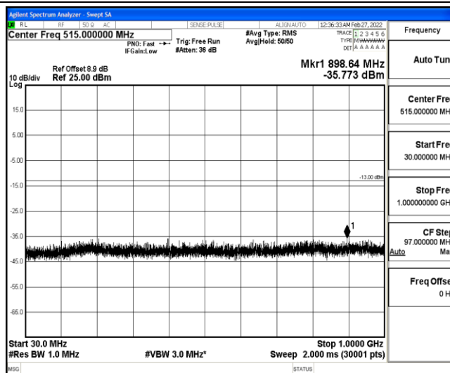
Band25-20MHz-QPSK-26365-1-0-Low-30-1000--35.77-PASS
