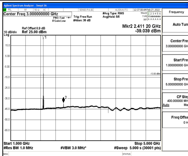
Band25-20MHz-QPSK-26365-1-0-Low-1000-5000--39.04-PASS
