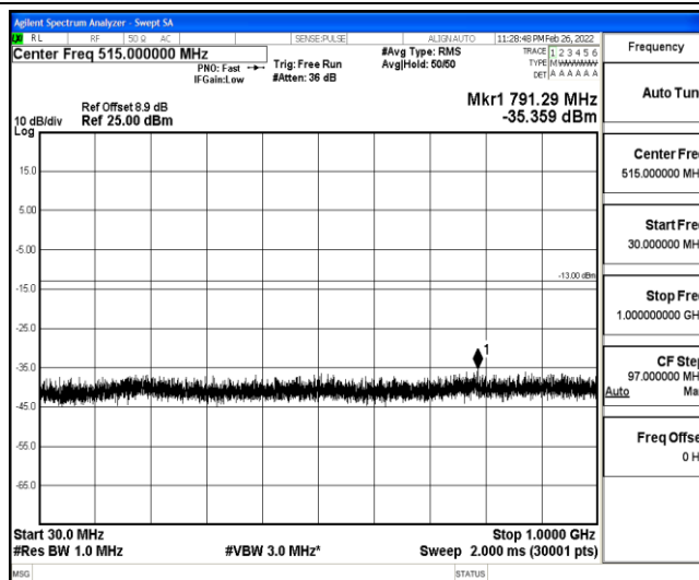
Band25-10MHz-QPSK-26365-1-0-Low-30-1000--35.36-PASS
