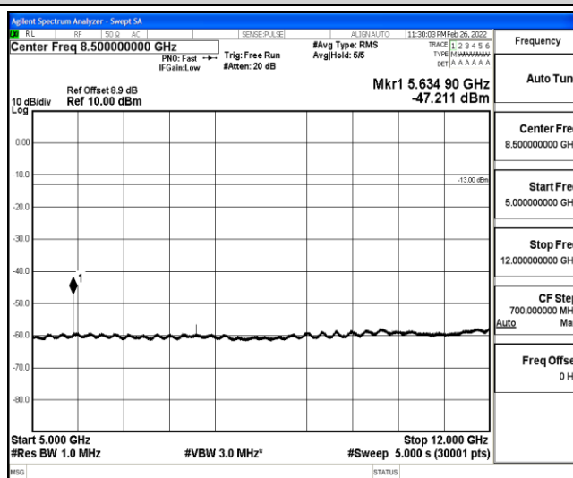
Band25-10MHz-QPSK-26365-1-0-Low-5000-12000--47.21-PASS
