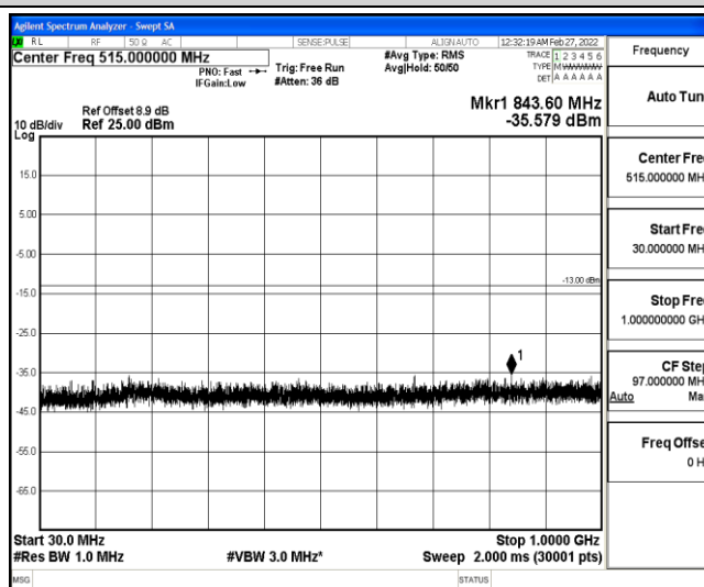
Band25-20MHz-QPSK-26140-1-0-Low-30-1000--35.58-PASS
