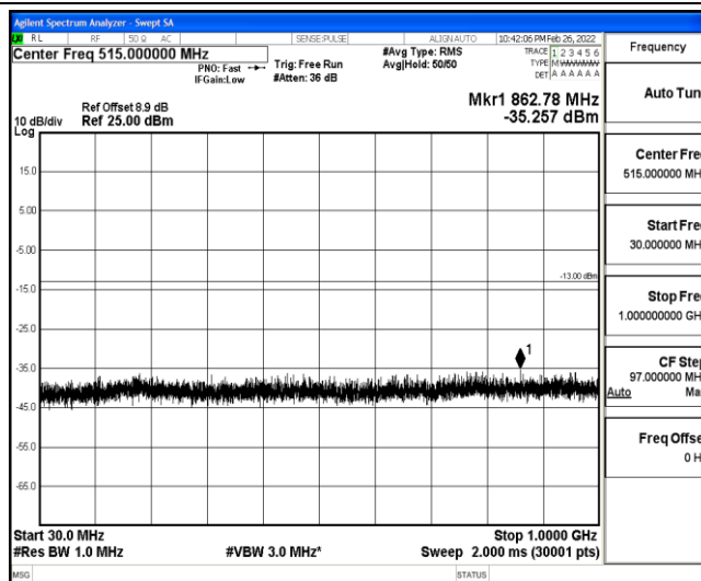
Band25-5MHz-QPSK-26365-1-0-Low-30-1000--35.26-PASS
