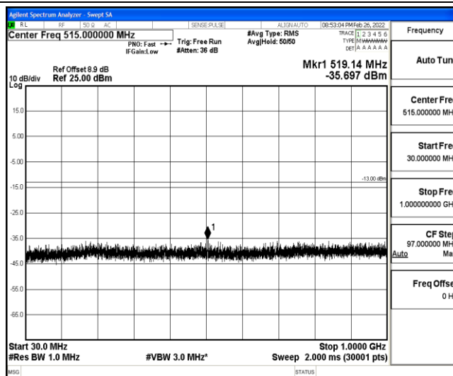
Band25-1.4MHz-QPSK-26365-1-0-Low-30-1000--35.7-PASS
