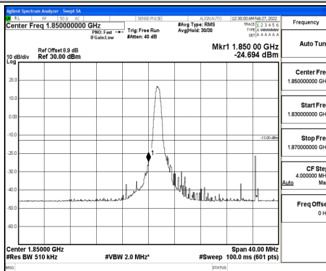
Band25-20MHz-QPSK-26140-1-0-Low--24.69-PASS
