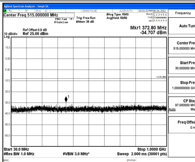
Band25-3MHz-QPSK-26365-1-0-Low-30-1000--34.71-PASS
