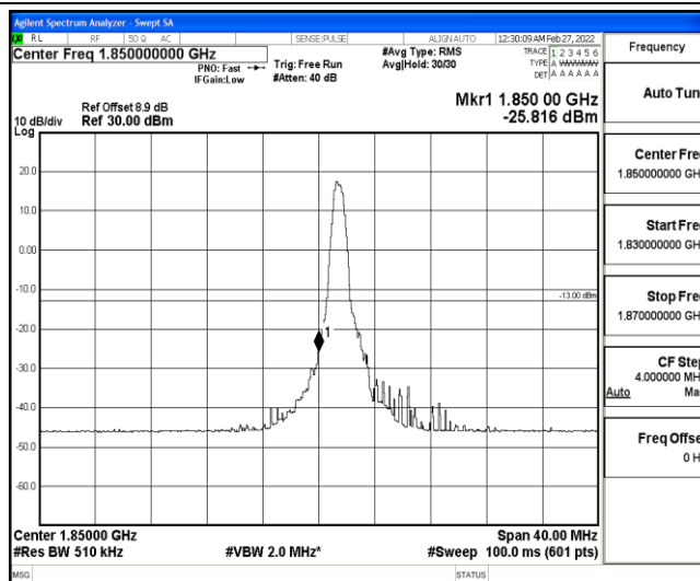
Band25-20MHz-16QAM-26140-1-0-Low--25.82-PASS
