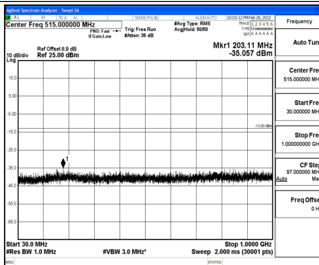
Band25-3MHz-16QAM-26365-1-0-Low-30-1000--35.06-PASS
