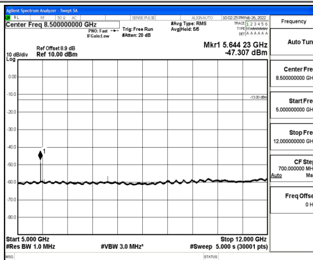
Band25-3MHz-QPSK-26365-1-0-Low-5000-12000--47.31-PASS
