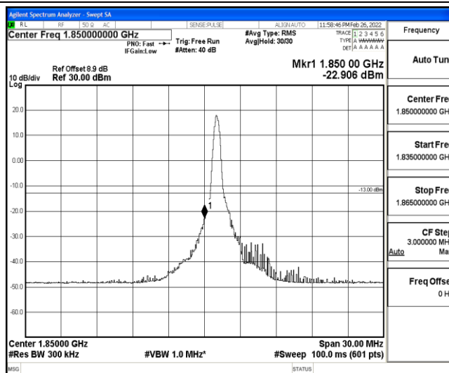
Band25-15MHz-QPSK-26115-1-0-Low--22.91-PASS
