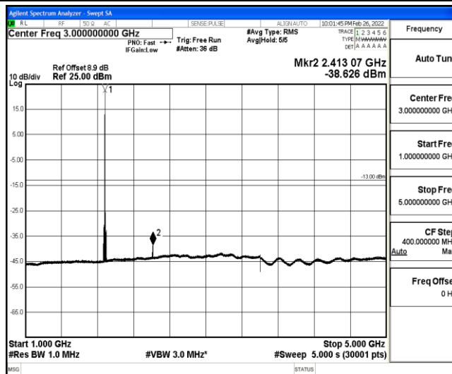
Band25-3MHz-QPSK-26365-1-0-Low-1000-5000--38.63-PASS
