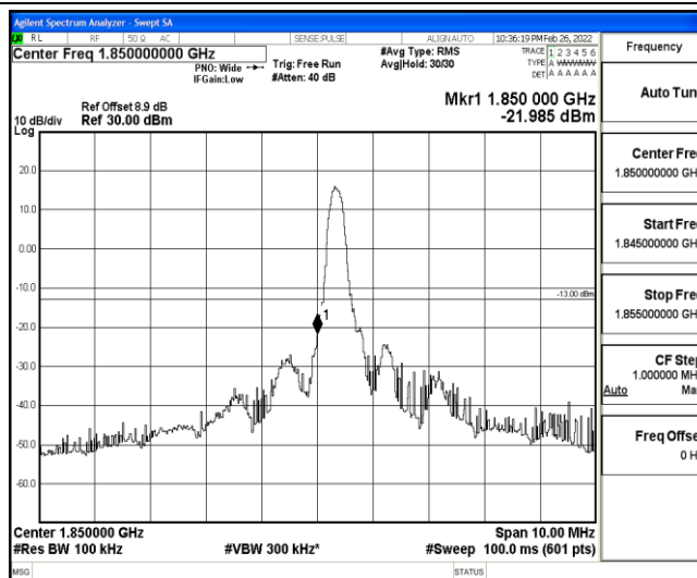
Band25-5MHz-16QAM-26065-1-0-Low--21.99-PASS
