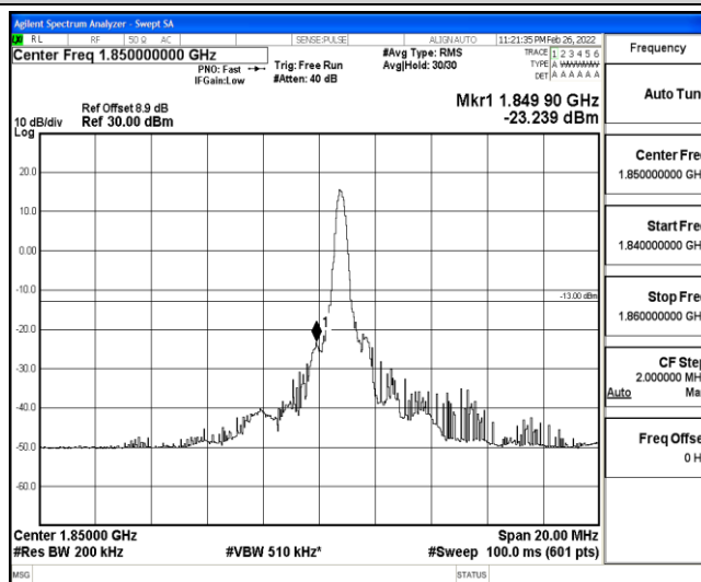
Band25-10MHz-16QAM-26090-1-0-Low--23.24-PASS
