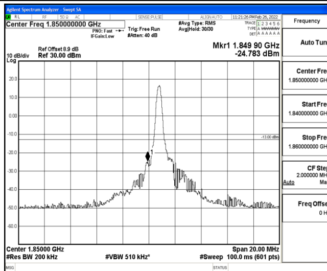
Band25-10MHz-QPSK-26090-1-0-Low--24.78-PASS
