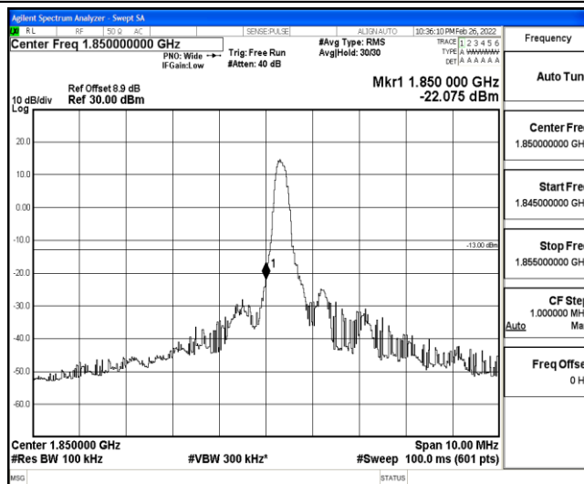
Band25-5MHz-QPSK-26065-1-0-Low--22.07-PASS
