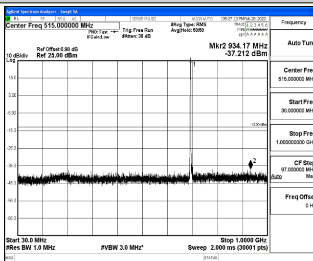
Band12-10MHz-QPSK-23060-1-0-Low-30-1000--37.21-PASS
