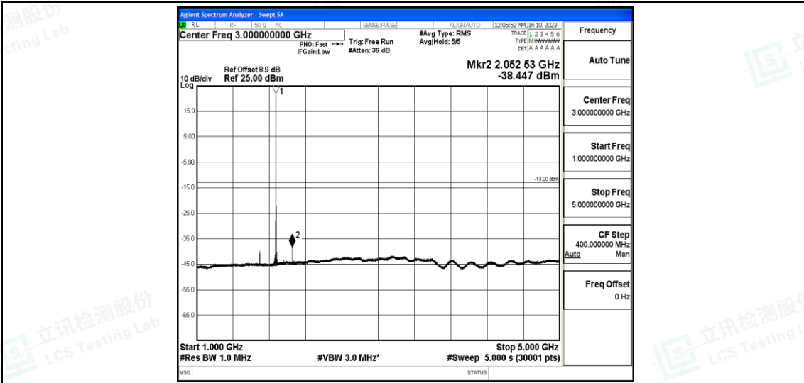
Band25-20MHz-16QAM-26365-1-0-Low-1000-5000--38.45-PASS
