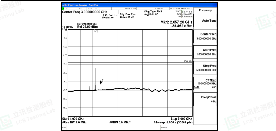
Band25-10MHz-QPSK-26365-1-0-Low-1000-5000--38.46-PASS
