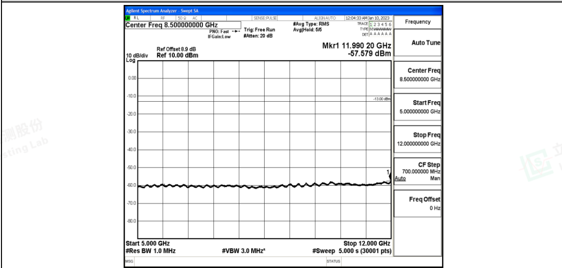
Band25-20MHz-QPSK-26365-1-0-Low-5000-12000--57.58-PASS
