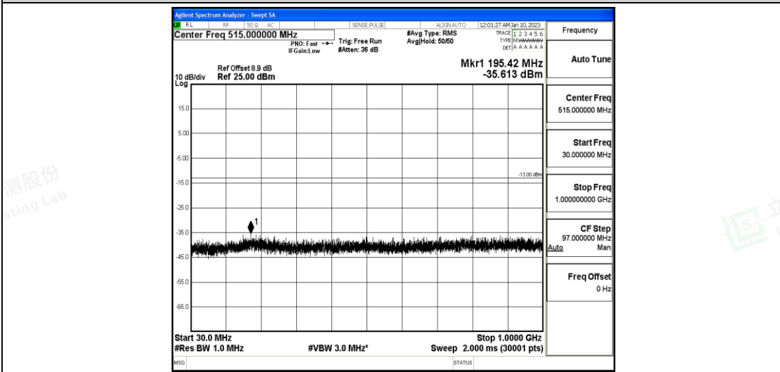
Band25-20MHz-16QAM-26140-1-0-Low-30-1000--35.61-PASS
