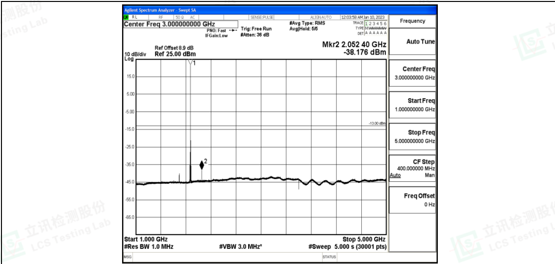
Band25-20MHz-QPSK-26365-1-0-Low-1000-5000--38.18-PASS
