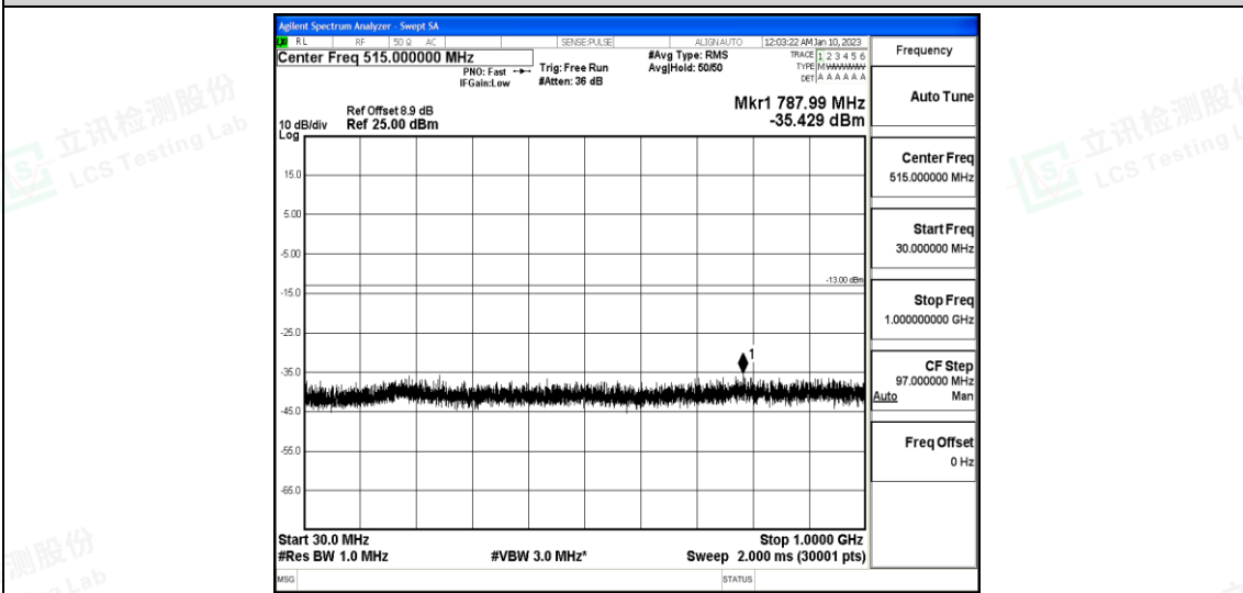
Band25-20MHz-QPSK-26365-1-0-Low-30-1000--35.43-PASS
