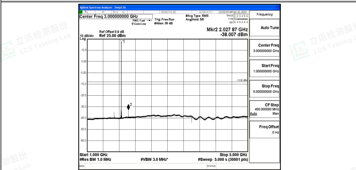
Band25-20MHz-16QAM-26140-1-0-Low-1000-5000--38.01-PASS
