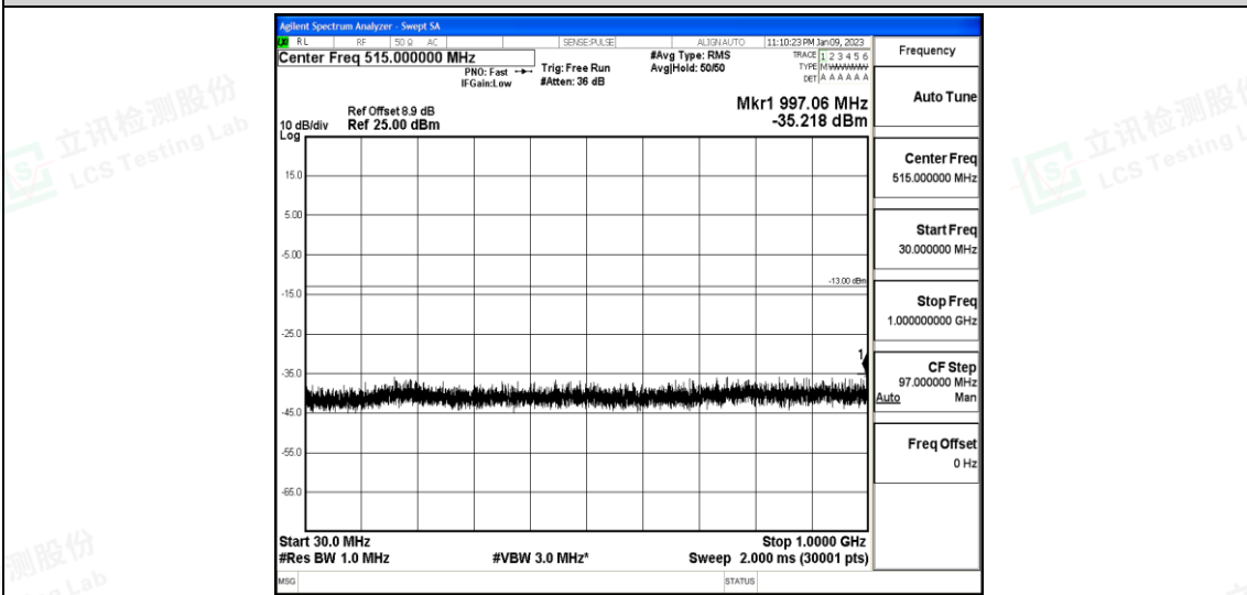
Band25-10MHz-QPSK-26365-1-0-Low-30-1000--35.22-PASS
