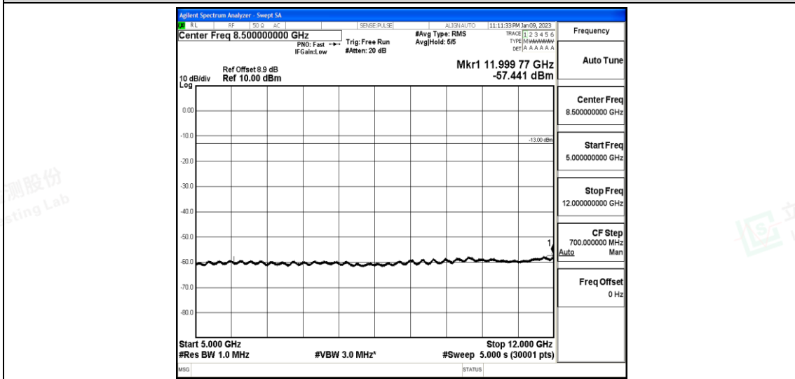
Band25-10MHz-QPSK-26365-1-0-Low-5000-12000--57.44-PASS
