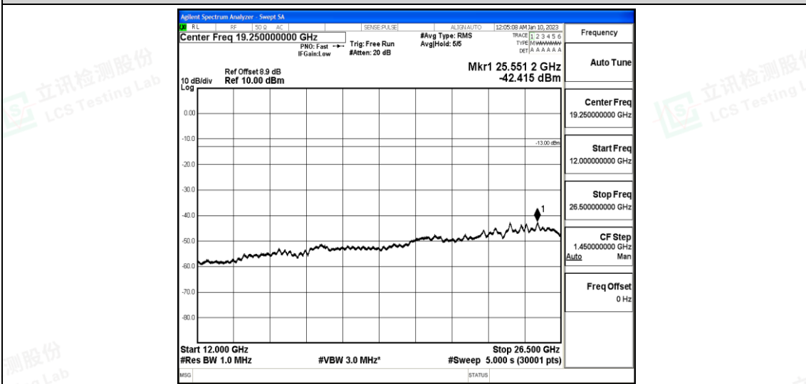
Band25-20MHz-QPSK-26365-1-0-Low-12000-26500--42.42-PASS
