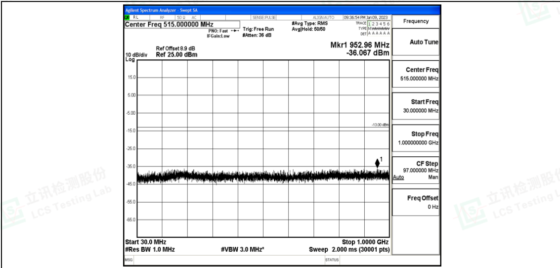
Band25-1.4MHz-QPSK-26047-1-0-Low-30-1000--36.07-PASS
