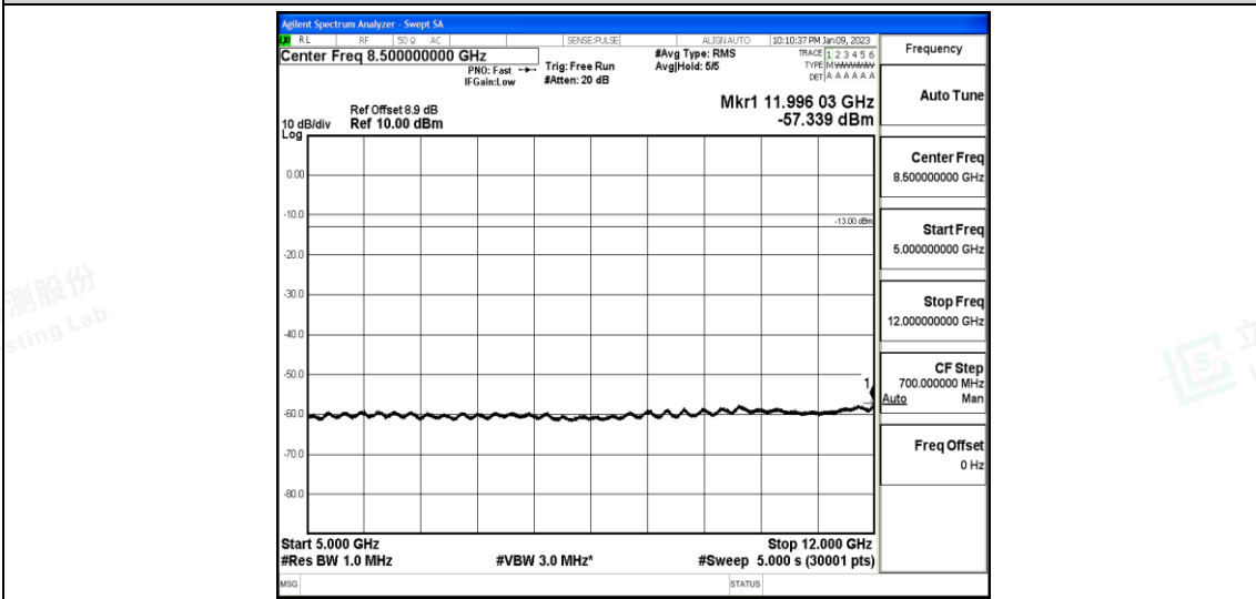
Band25-3MHz-QPSK-26365-1-0-Low-5000-12000--57.34-PASS
