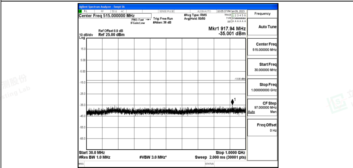
Band25-3MHz-QPSK-26055-1-0-Low-30-1000--35-PASS
