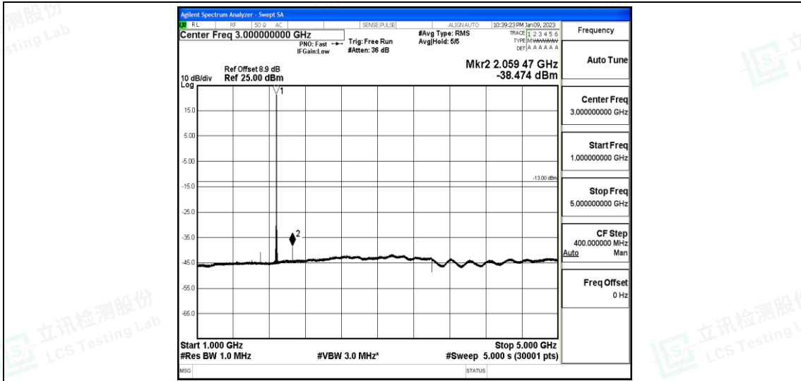
Band25-5MHz-QPSK-26365-1-0-Low-1000-5000--38.47-PASS
