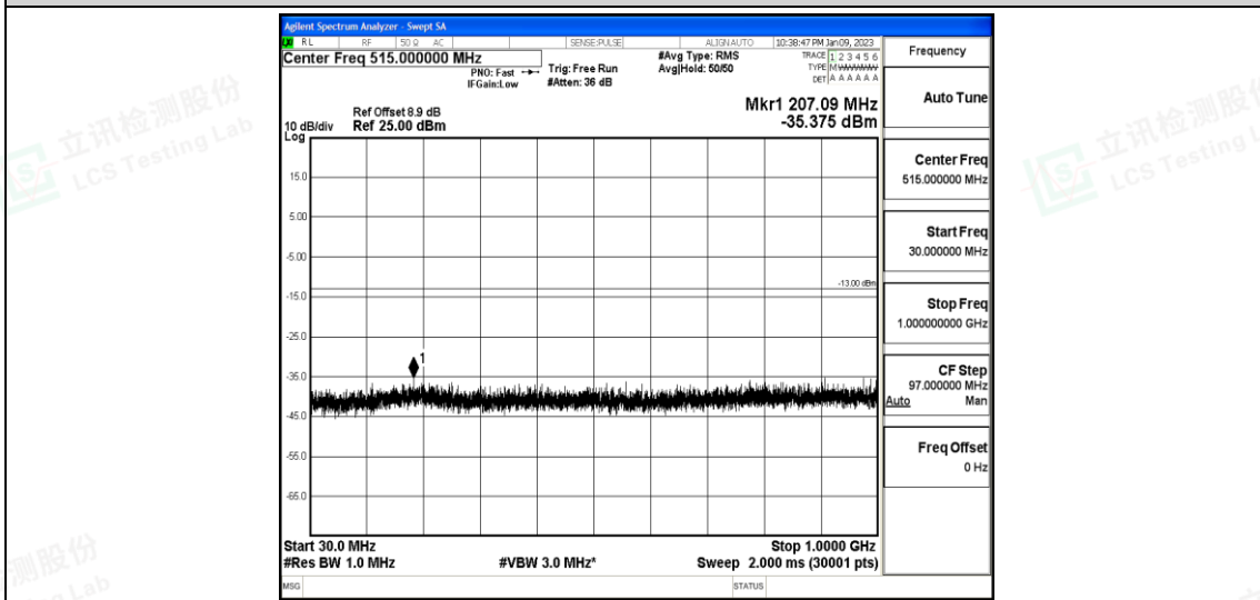
Band25-5MHz-QPSK-26365-1-0-Low-30-1000--35.38-PASS
