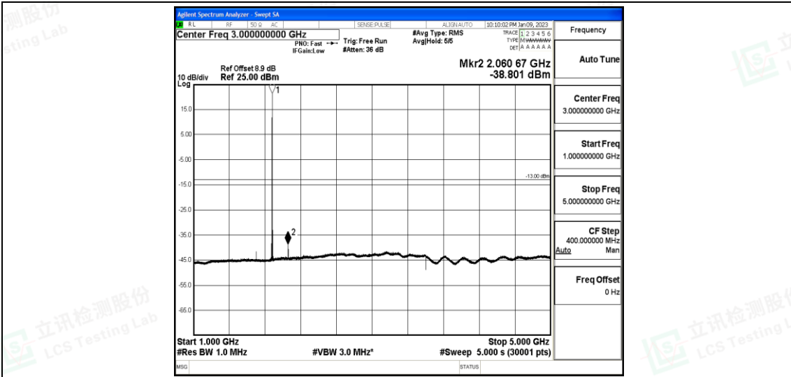
Band25-3MHz-QPSK-26365-1-0-Low-1000-5000--38.8-PASS
