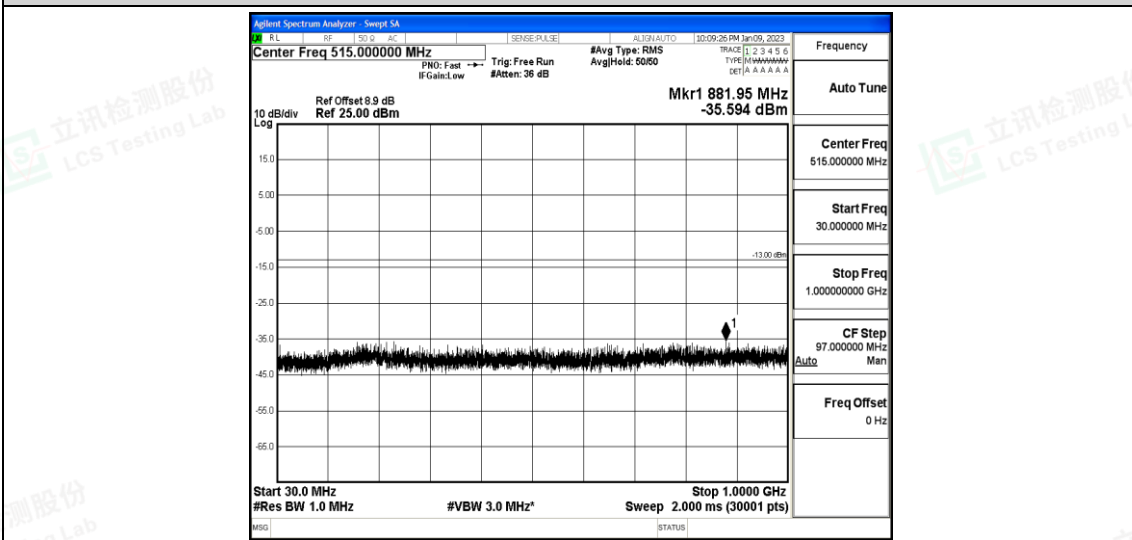
Band25-3MHz-QPSK-26365-1-0-Low-30-1000--35.59-PASS
