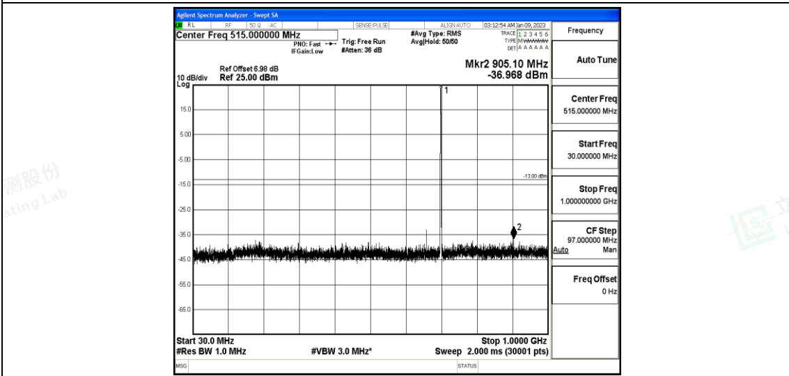
Band12-3MHz-QPSK-23095-1-0-Low-30-1000--36.97-PASS
