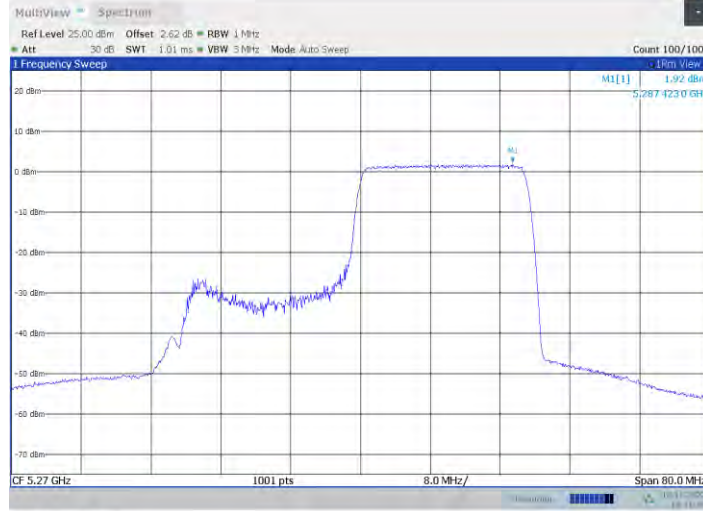
11ax40MIMO_Ant4_5270_242Tone_RU61
