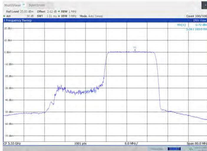
11ax40MIMO_Ant4_5550_242Tone_RU62
