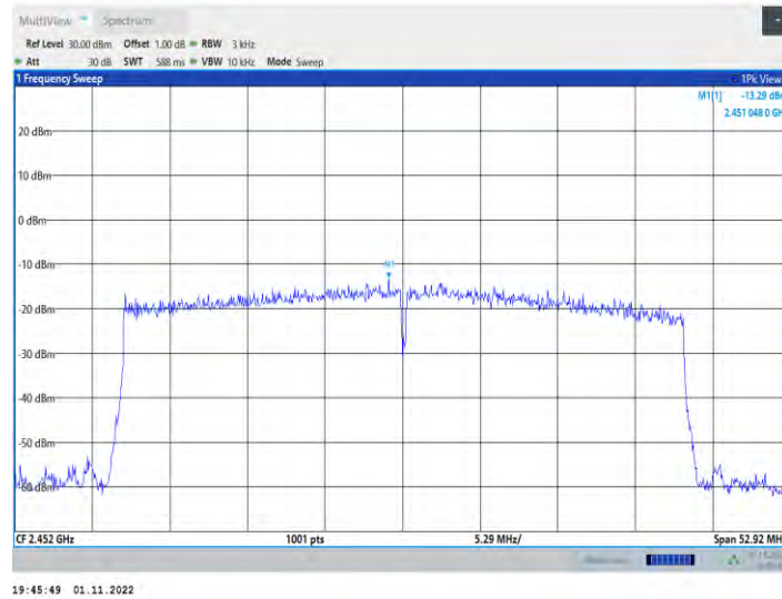
11ax40MIMO_Ant2_2452
