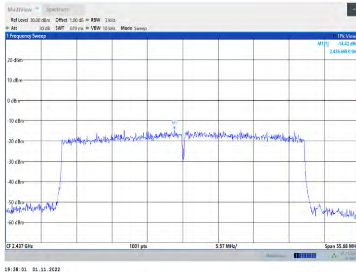
11ax40MIMO_Ant4_2437
