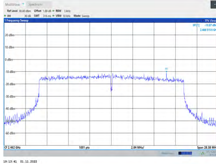
11ax20MIMO_Ant4_2462
