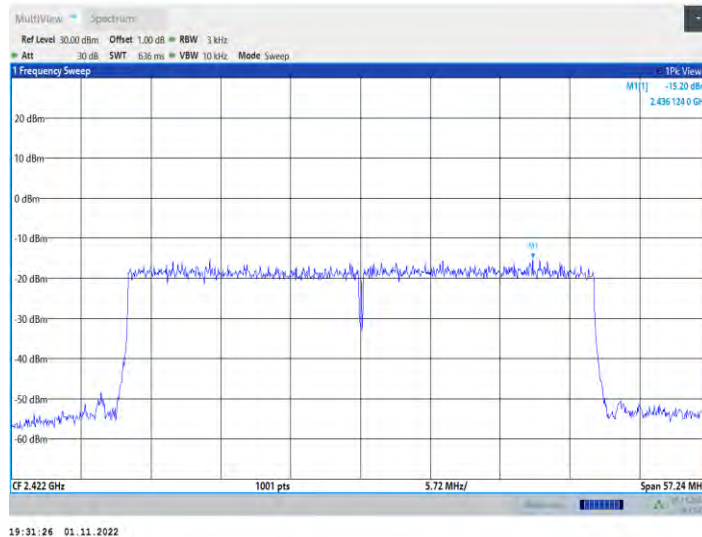
11ax40MIMO_Ant4_2422
