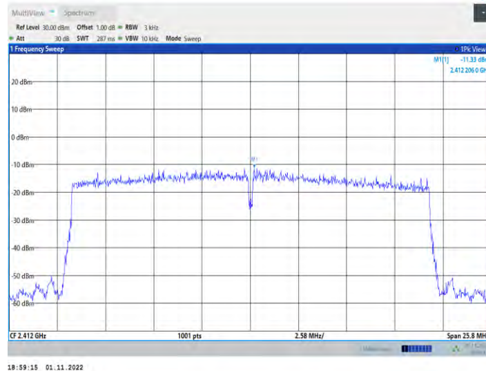
11ax20MIMO_Ant4_2412
