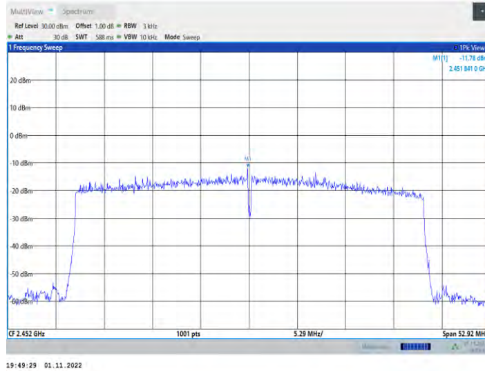
11ax40MIMO_Ant4_2452
