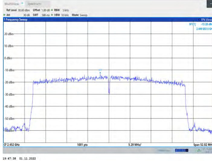
11ax40MIMO_Ant4_2452
