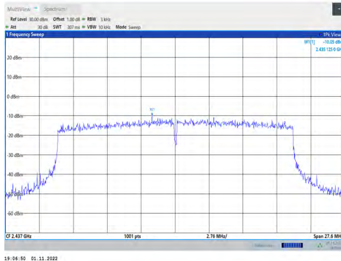
11ax20MIMO_Ant4_2437
