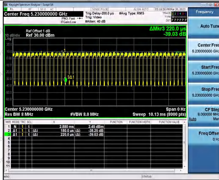
11N40SISO_Ant2_5230
