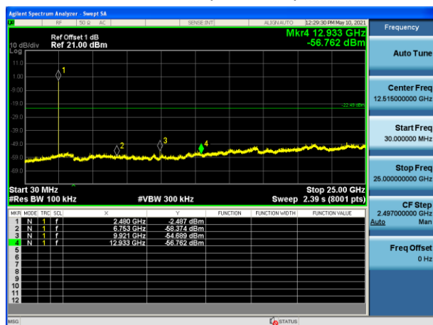
Mode 2/ CH78(2480MHz)
