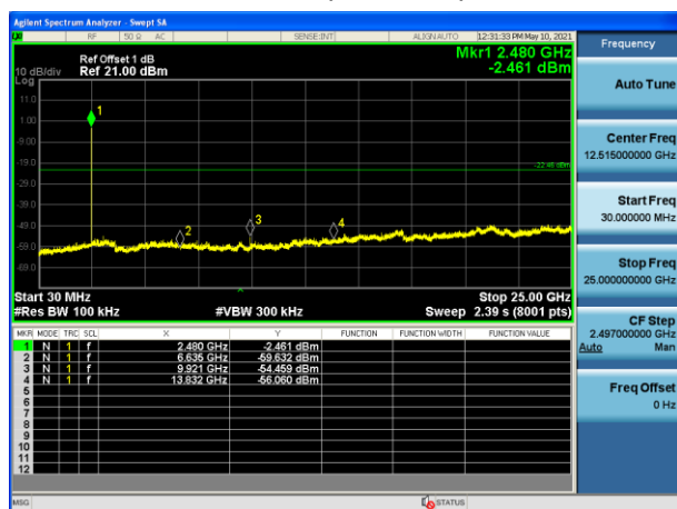
Mode 3/ CH78(2480MHz)
