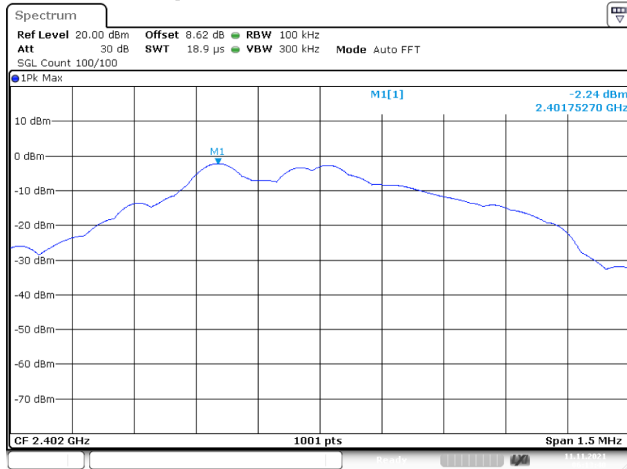
T Tx. Spurious NVNT BLE 1M 2402MHz Ant1 Ref
