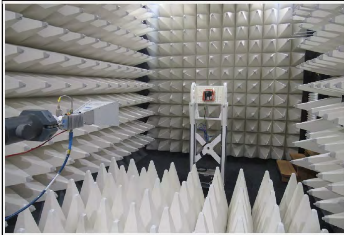
Setup 8-18GHz
