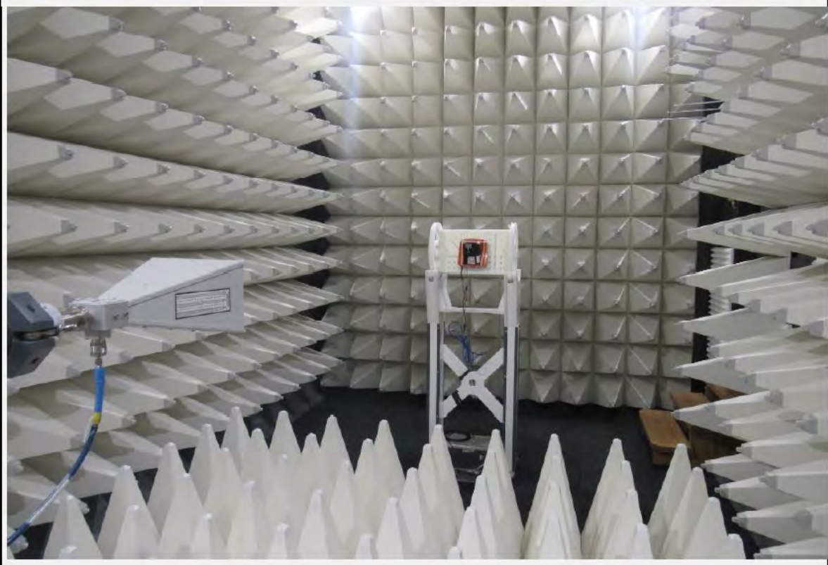
Setup 1-8GHz
