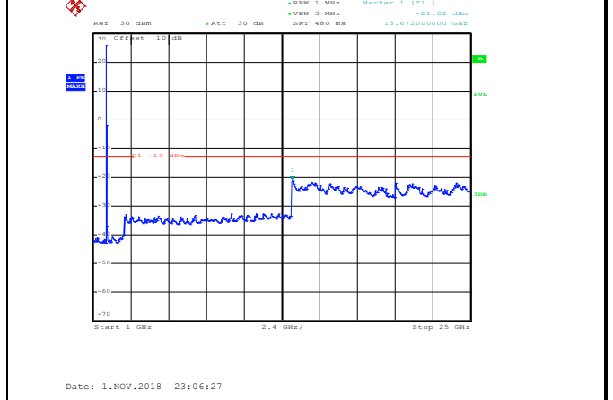
1GHz~25GHz
