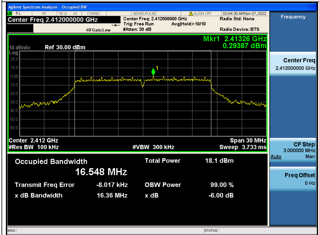
Test_Graph_802.11g_ANT1_2412_6Mbps_DTBSW
