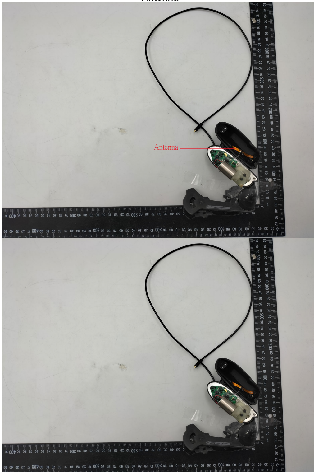
Antenna
