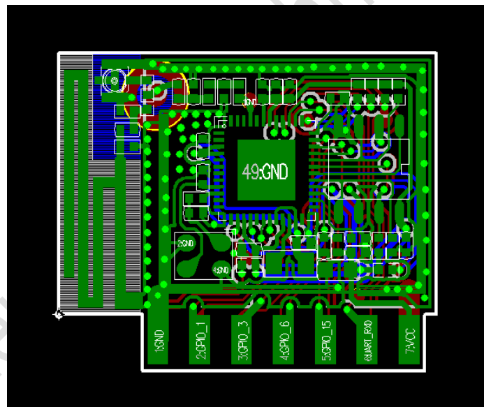
Figure 3 UA504module exterior
