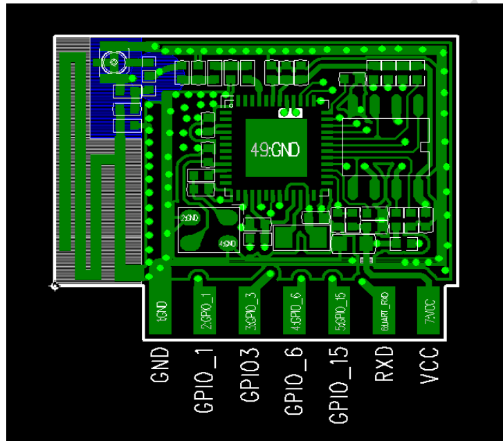
Figure 1 UA504 top layer
