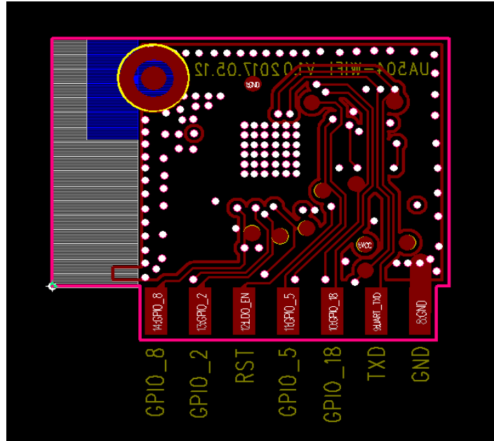
Figure 2 UA504 bottom layer
