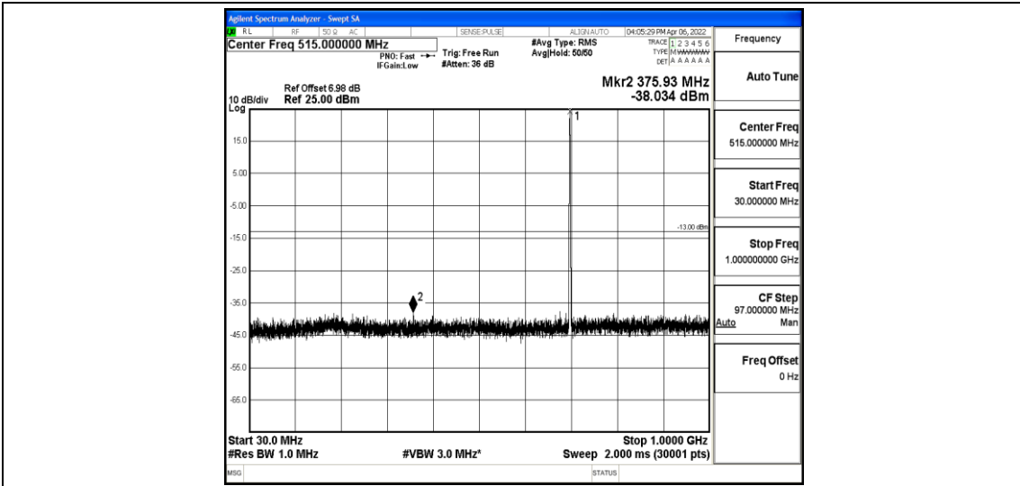
Band12-5MHz-QPSK-23095-1-0-Low-30-1000--38.03-PASS
