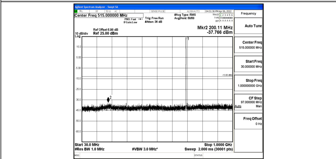
Band12-5MHz-QPSK-23035-1-0-Low-30-1000--37.77-PASS
