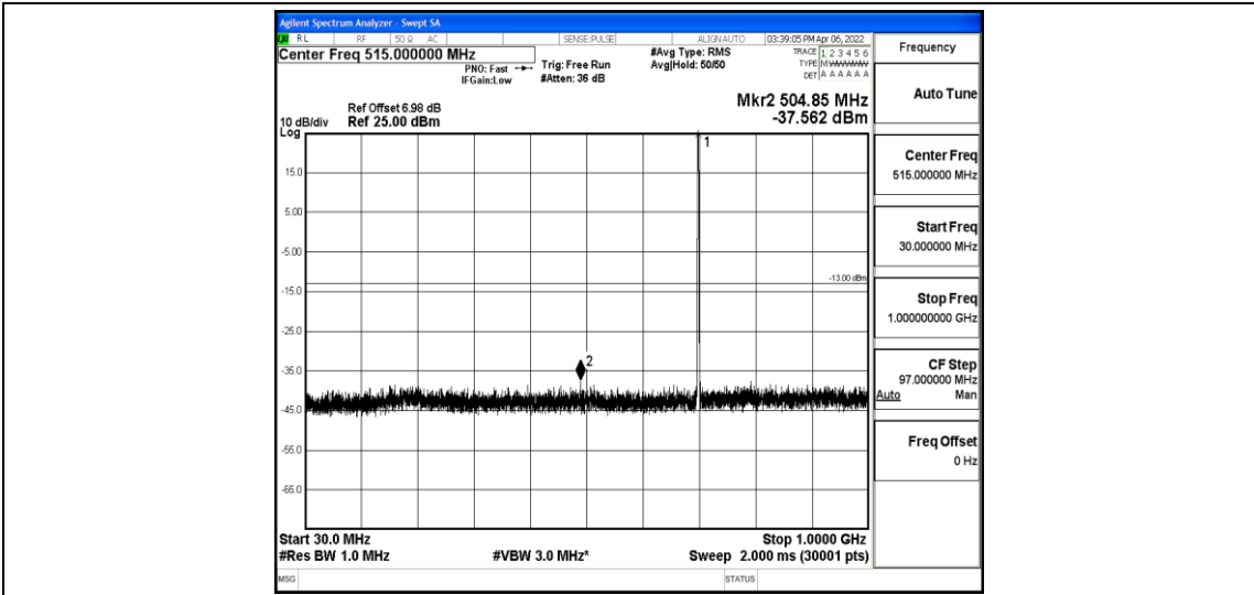
Band12-3MHz-16QAM-23095-1-0-Low-30-1000--37.56-PASS
