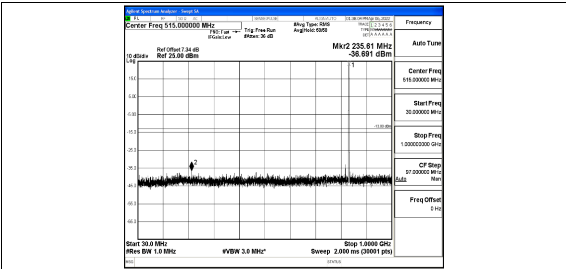
Band5-3MHz-16QAM-20525-1-0-Low-30-1000--36.69-PASS
