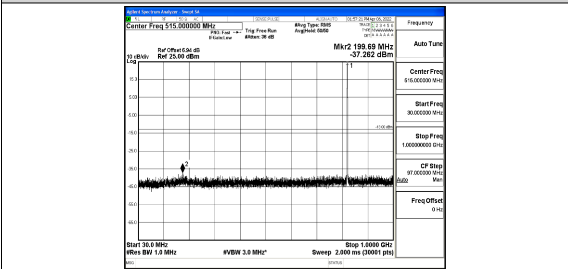
Band5-5MHz-QPSK-20425-1-0-Low-30-1000--37.26-PASS
