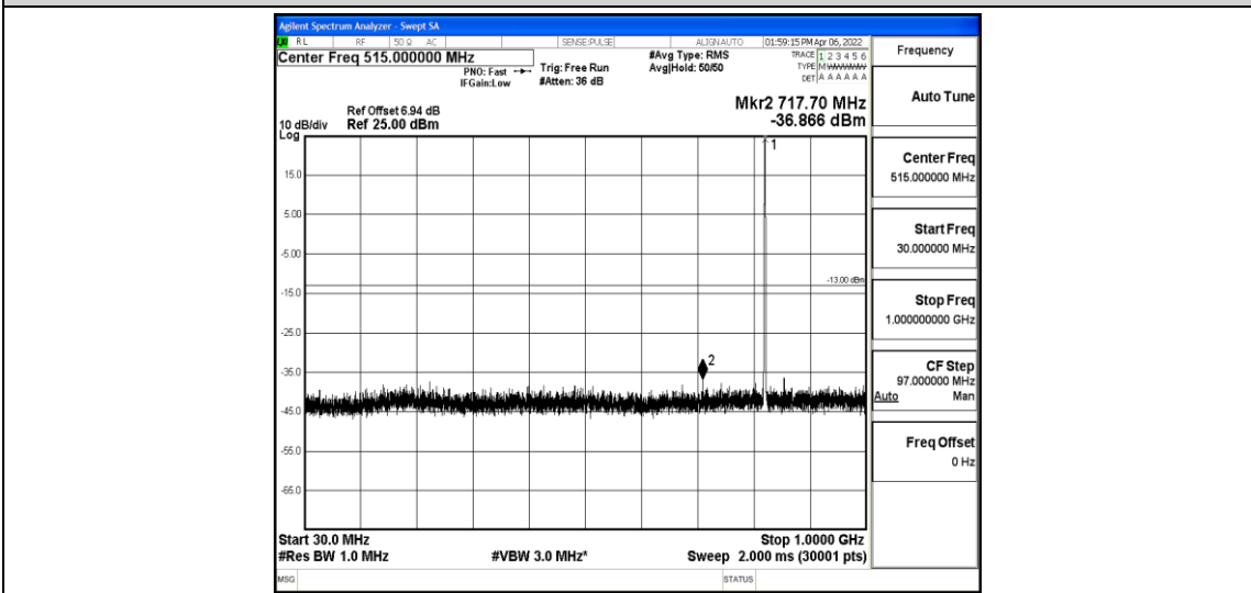
Band5-5MHz-16QAM-20425-1-0-Low-30-1000--36.87-PASS
