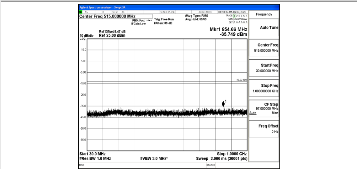
Band4-10MHz-QPSK-20000-1-0-Low-30-1000--35.75-PASS
