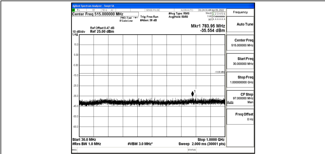
Band4-5MHz-QPSK-20175-1-0-Low-30-1000--35.55-PASS
