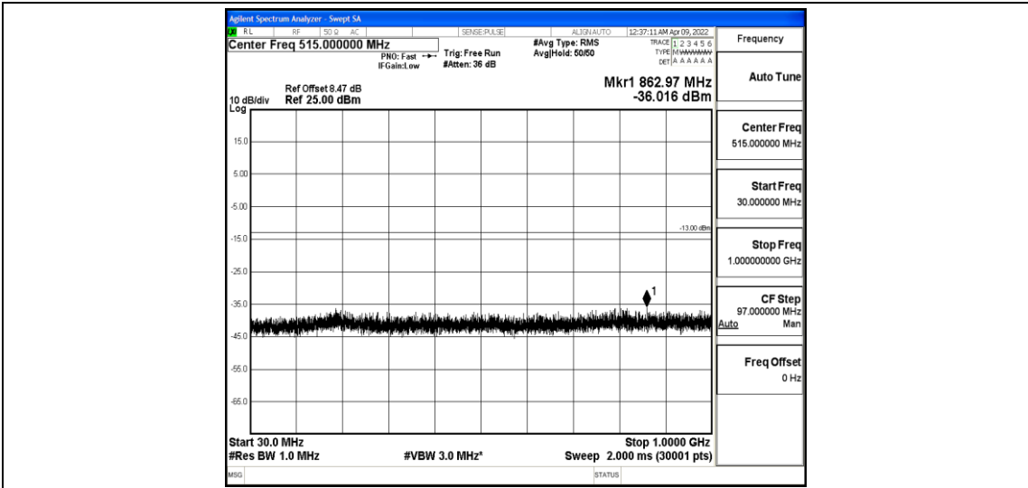
Band4-1.4MHz-QPSK-20175-1-0-Low-30-1000--36.02-PASS
