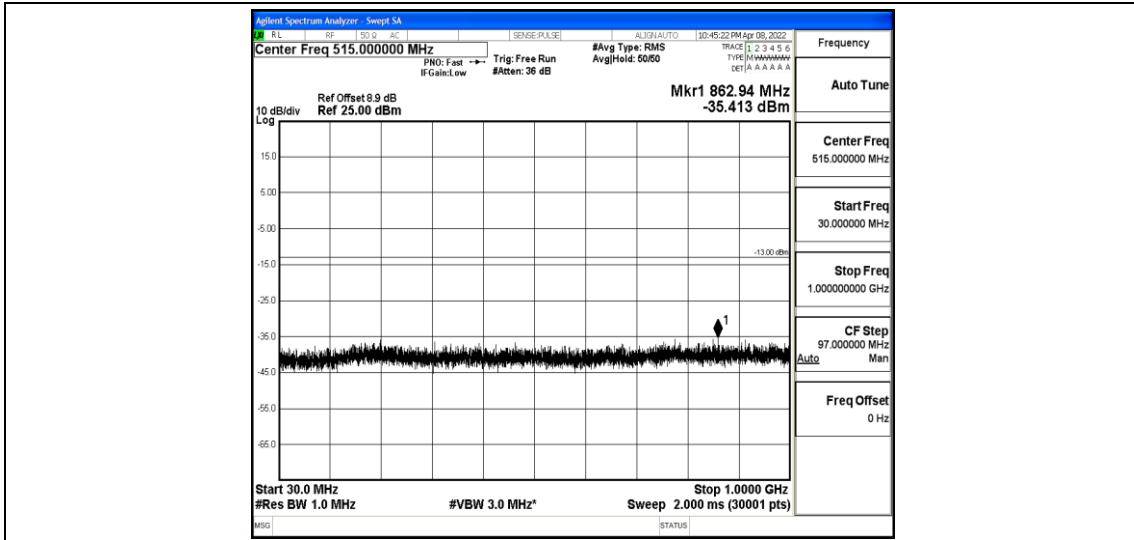
Band2-10MHz-QPSK-18900-1-0-Low-30-1000--35.41-PASS
