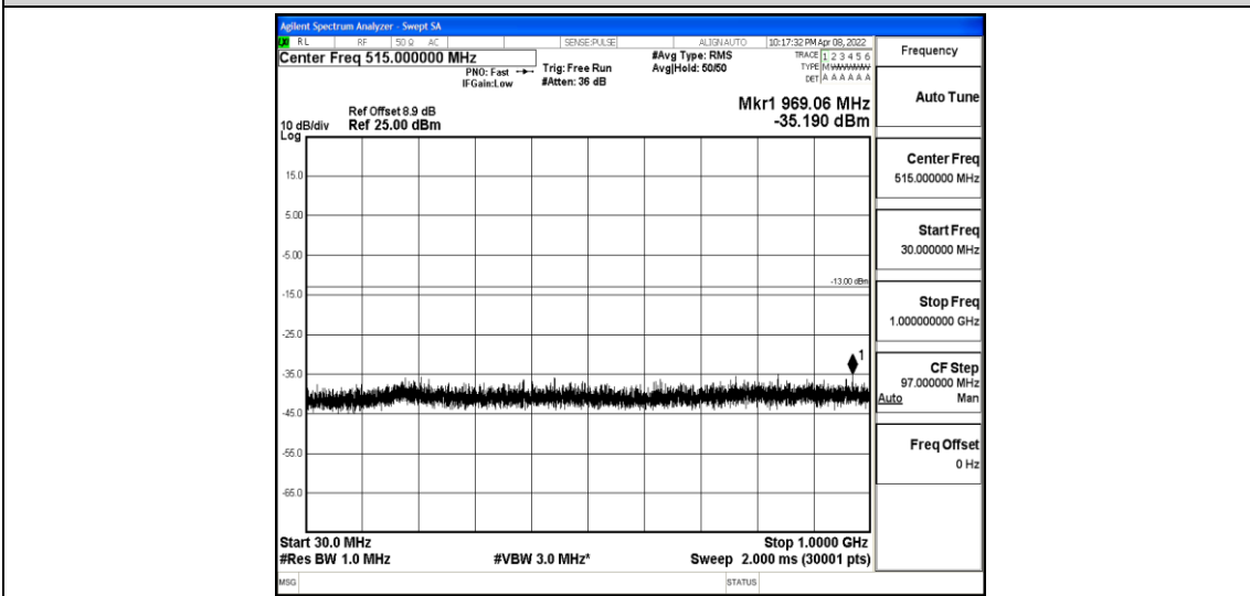
Band2-5MHz-QPSK-18625-1-0-Low-30-1000--35.19-PASS
