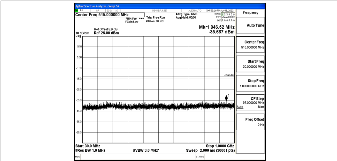
Band2-3MHz-16QAM-18900-1-0-Low-30-1000--35.67-PASS
