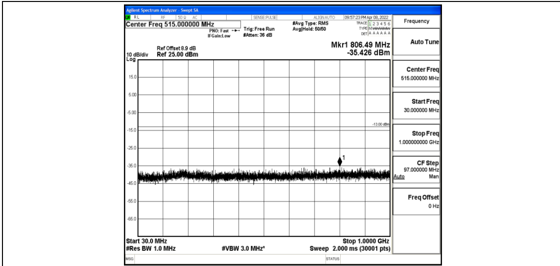
Band2-3MHz-QPSK-18900-1-0-Low-30-1000--35.43-PASS
