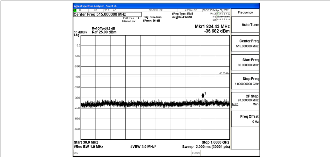
Band2-1.4MHz-QPSK-18900-1-0-Low-30-1000--35.68-PASS
