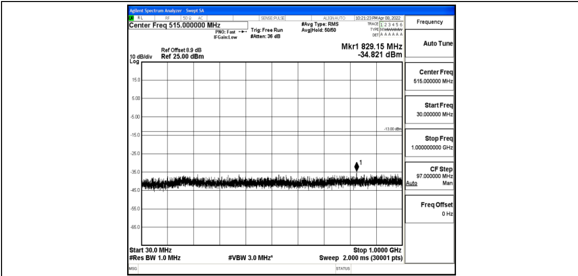
Band2-5MHz-QPSK-18900-1-0-Low-30-1000--34.82-PASS
