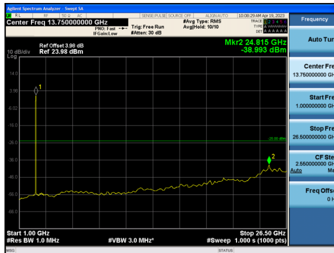
Band41-10MHz-QPSK-40690-1RB#0-Range2:1000~26500MHz
