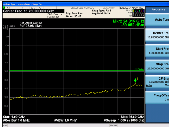
Band41-5MHz-QPSK-40690-1RB#0-Range2:1000~26500MHz
