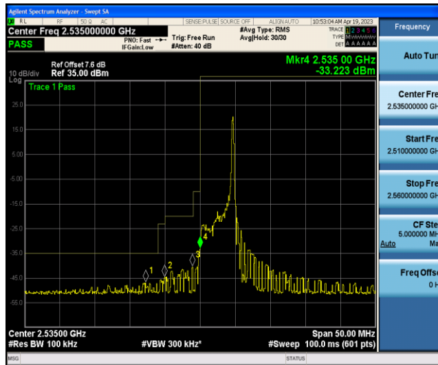
Band41-5MHz-QPSK-40065-25RB#0
