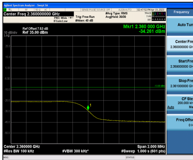
Band40-5MHz-QPSK-39225-1RB#24
