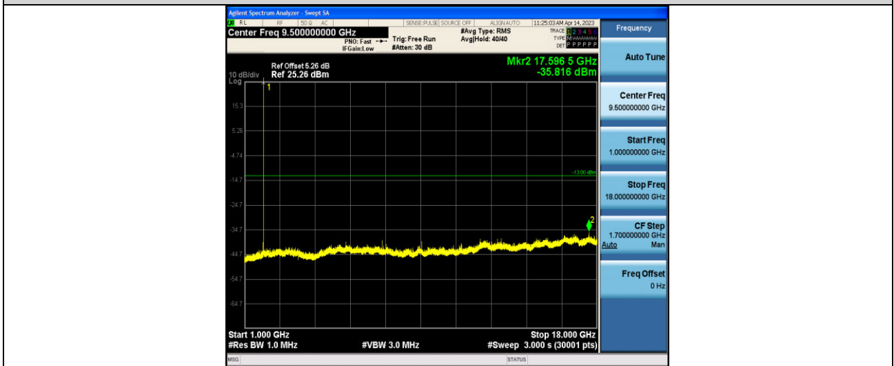
GPRS1900-810-1000~18000MHz
