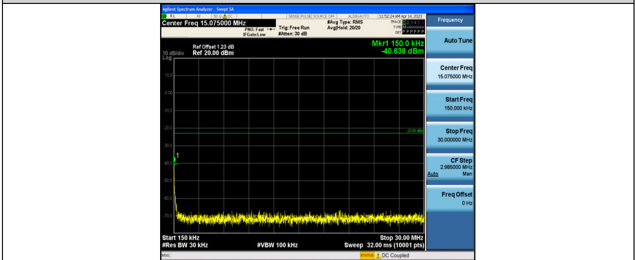
EGPRS1900-810-0.15~30MHz
