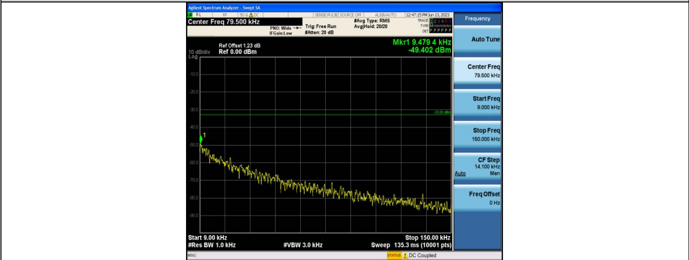
GPRS850-190-0.009~0.15MHz
