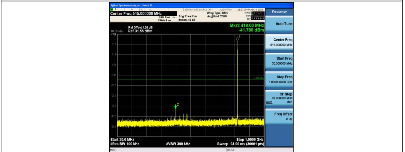
EGPRS850-128-30~1000MHz
