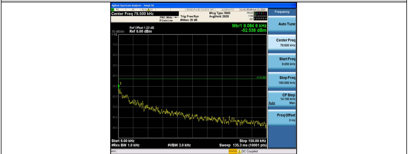
GPRS1900-512-0.009~0.15MHz
