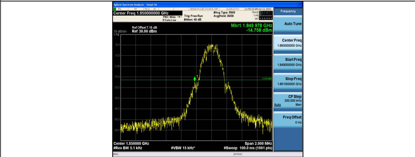
GPRS1900-512
