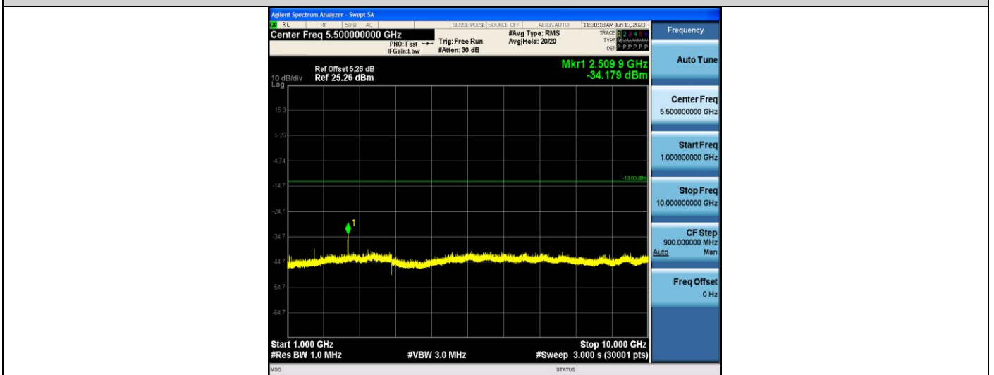
EGPRS850-190-1000~10000MHz
