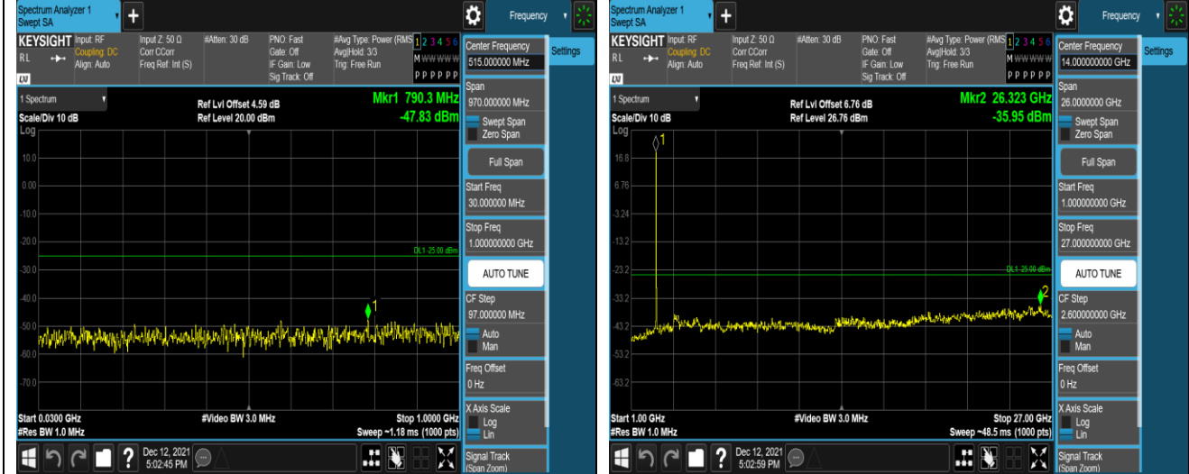
Band7-20MHz-QPSK-21100-1RB#0- Range1:30~1000MHz Band7-20MHz-QPSK-21100-1RB#0- Range2:1000~27000MHz
