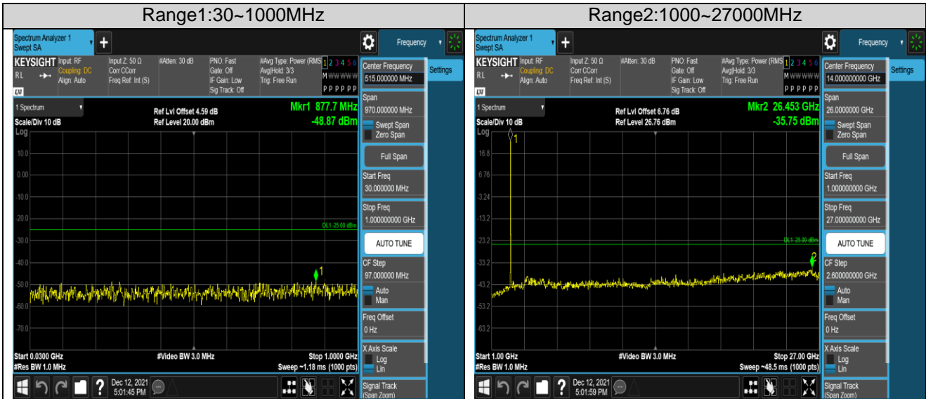
Band7-20MHz-QPSK-20850-1RB#0- Range1:30~1000MHz Band7-20MHz-QPSK-20850-1RB#0- Range2:1000~27000MHz
