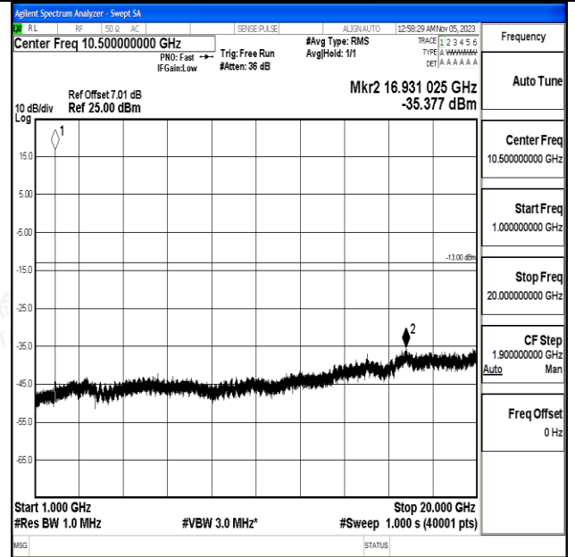
1 GHz – 20 GHz
