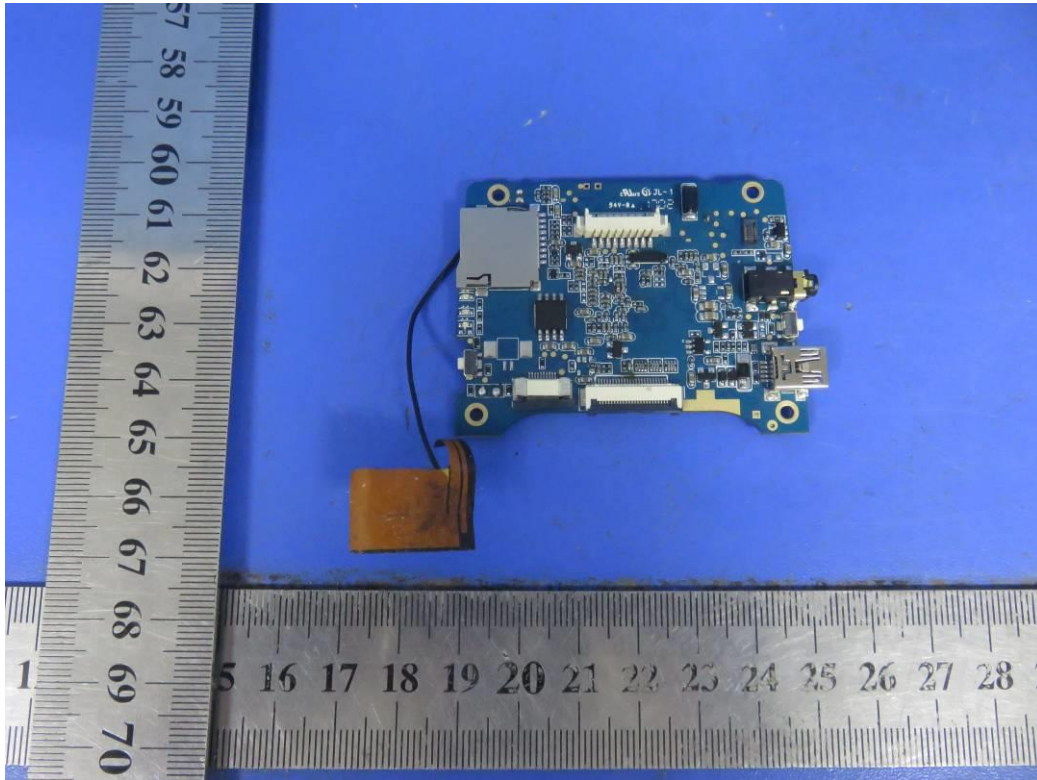
Fig.3 A305_PCB_Back
