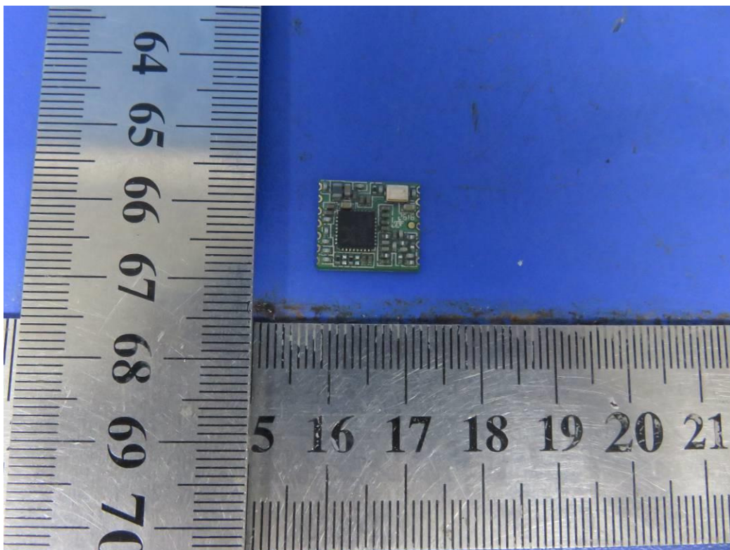
Fig.4 A305_WIFI Module_Front
