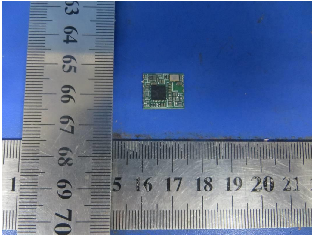
Fig.9 A307_WIFI Module_Front
