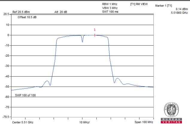
802.11ac (40MHz)_Chain 3 / CH102
