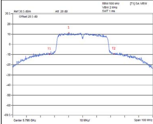
802.11ac(40MHz) Chain0 / CH159
