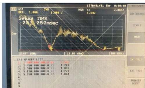
Aux - VSWR
