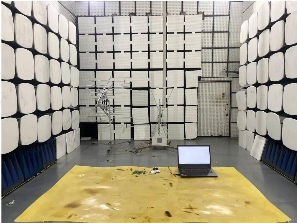
Fig. 2 (30MHz~1GHz)
