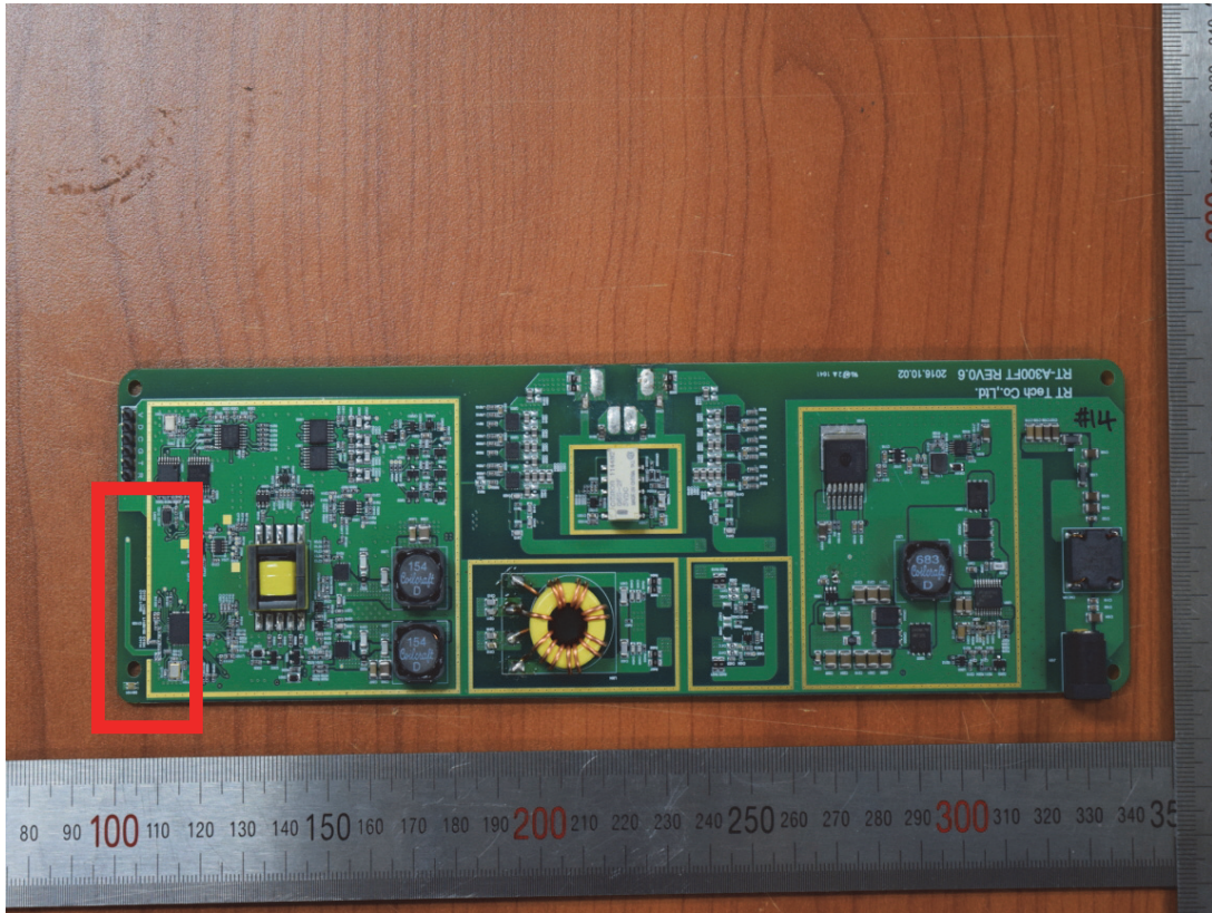
BLE Antenna
