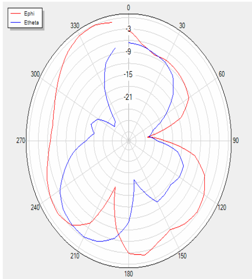
H Theta=90 freq=2420MHz
