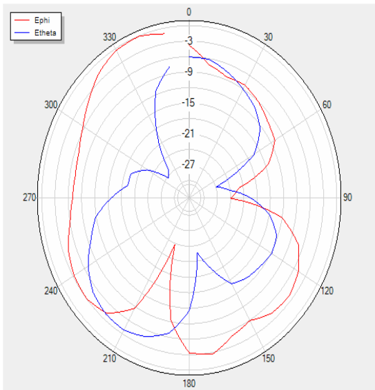
H Theta=90 freq=2420MHz
