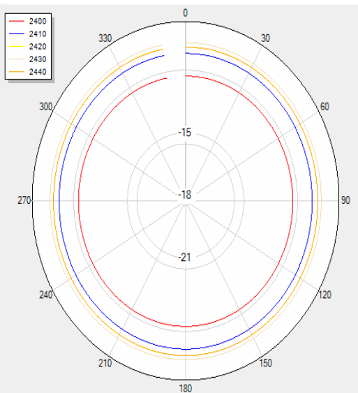
H Theta=0
