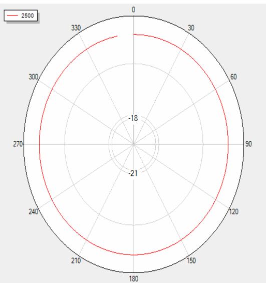
H Theta=0
