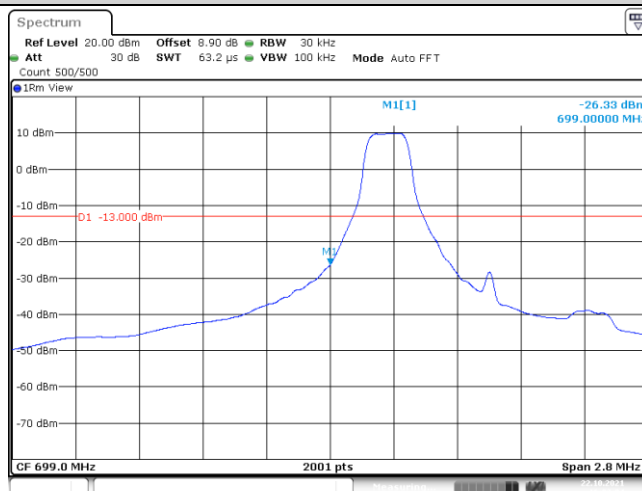
Band12-1.4MHz-16QAM-23017-1-0-Low--26.33-PASS
