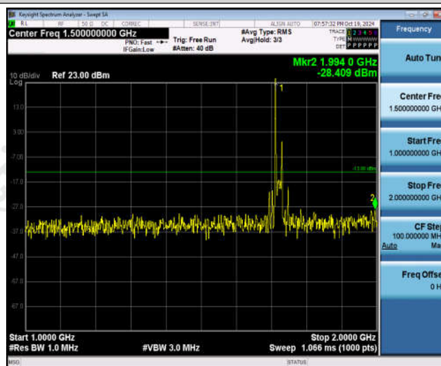
Band66-20MHz-QPSK-132072-1RB#0-Range2:1000~2000MHz
