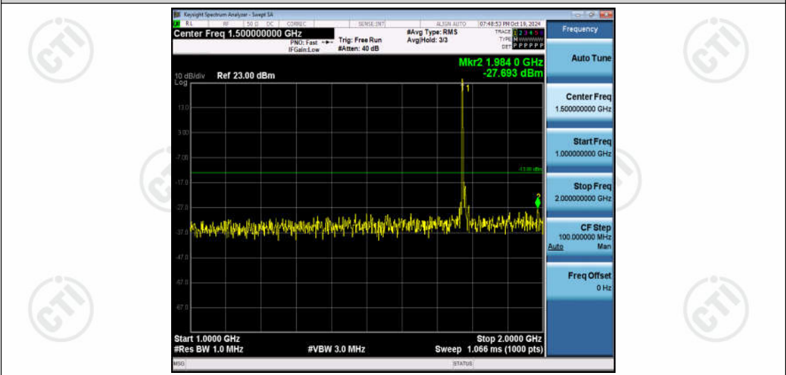
Band66-10MHz-QPSK-132622-1RB#0-Range2:1000~2000MHz
