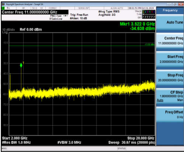
Band66-20MHz-QPSK-132572-1RB#0-Range3:2000~20000MHz
