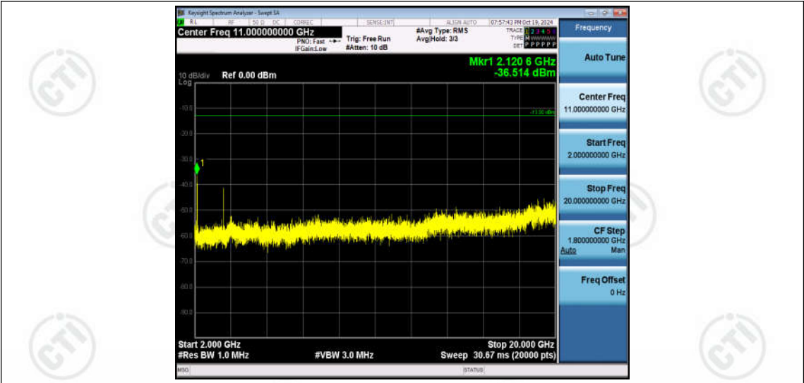
Band66-20MHz-QPSK-132072-1RB#0-Range3:2000~20000MHz
