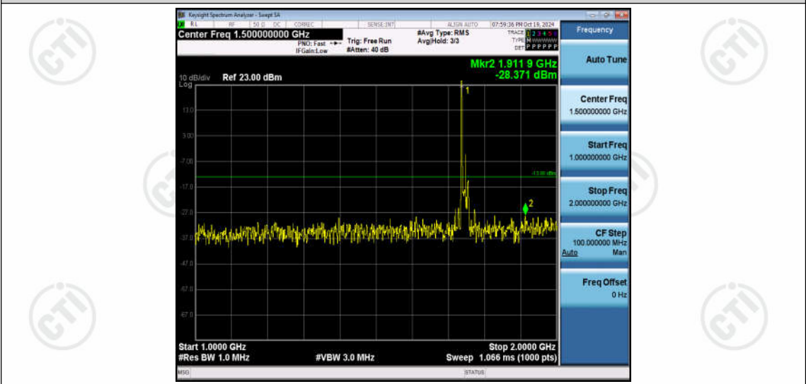
Band66-20MHz-QPSK-132322-1RB#0-Range2:1000~2000MHz
