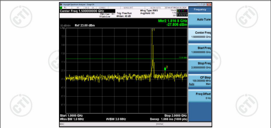
Band66-10MHz-QPSK-132022-1RB#0-Range2:1000~2000MHz
