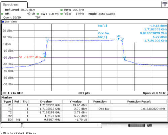
Band66-10MHz-QPSK-132022-50RB#0-9.018
