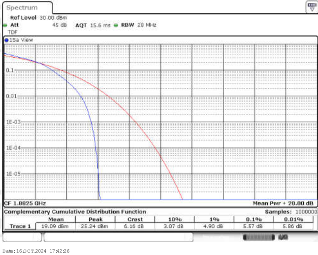
Band25-20MHz-16QAM-26365-25RB#0
