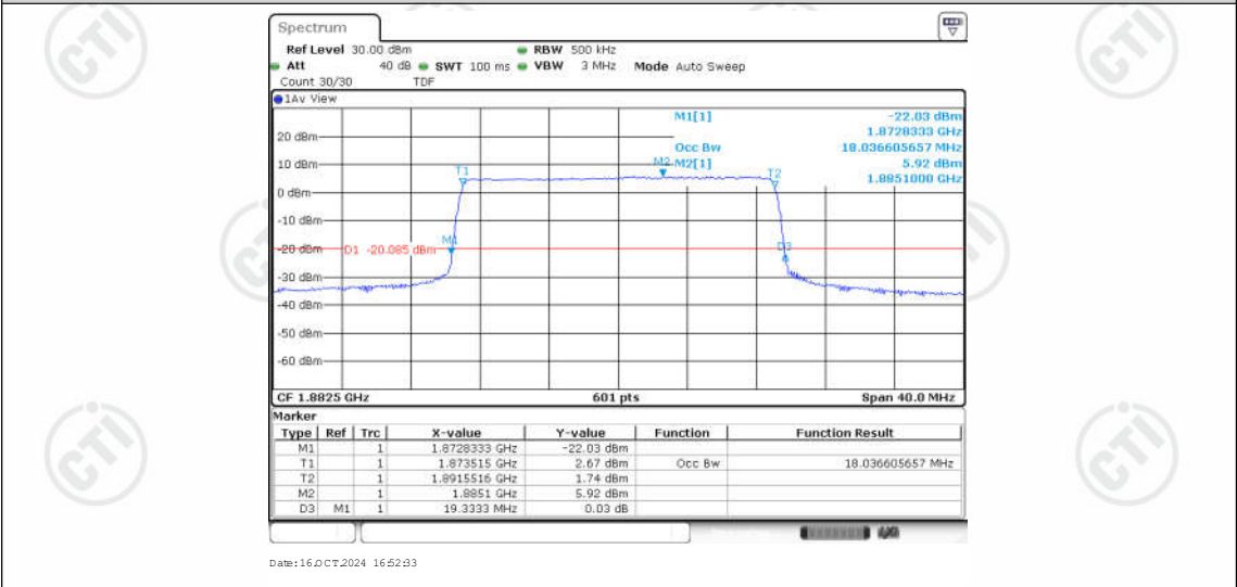
Band25-20MHz-QPSK-26365-100RB#0-18.037
