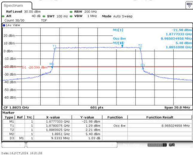
Band25-10MHz-QPSK-26365-50RB#0-8.985
