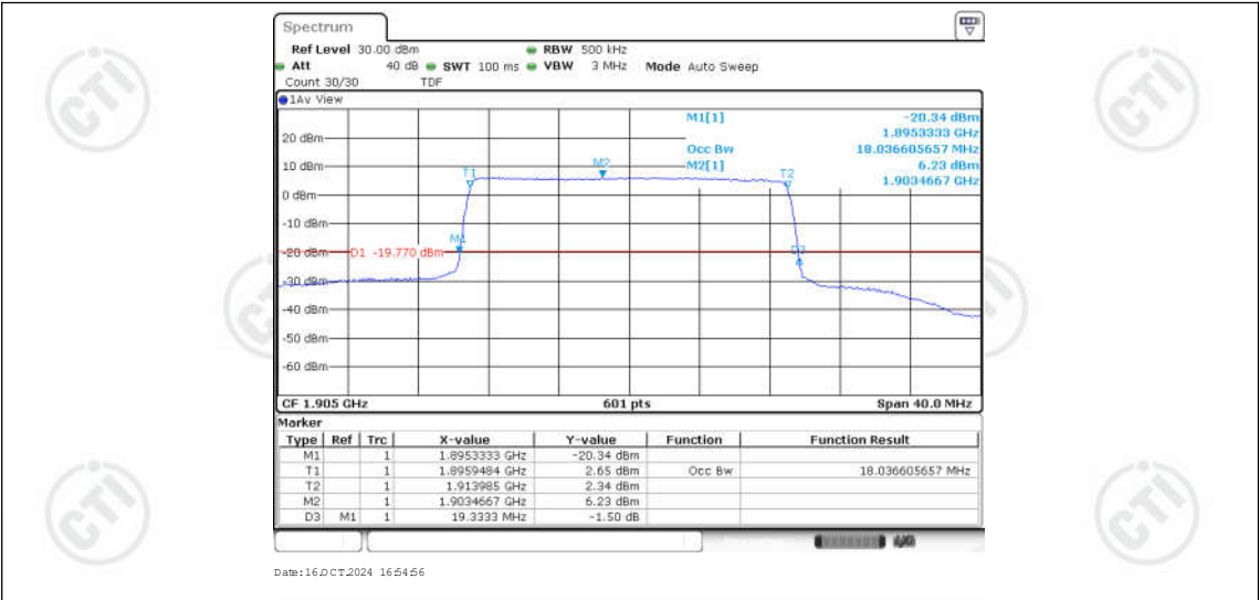
Band25-20MHz-QPSK-26590-100RB#0-18.037
