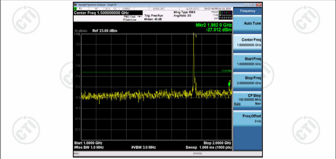
Band4-10MHz-QPSK-20350-1RB#0-Range2:1000~2000MHz
