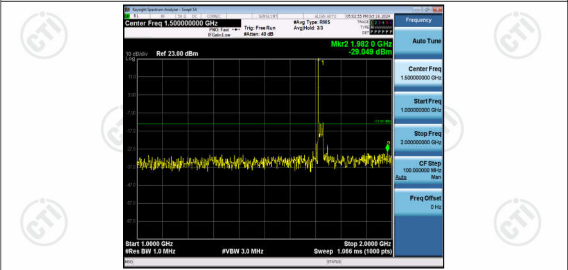
Band4-20MHz-QPSK-20050-1RB#0-Range2:1000~2000MHz
