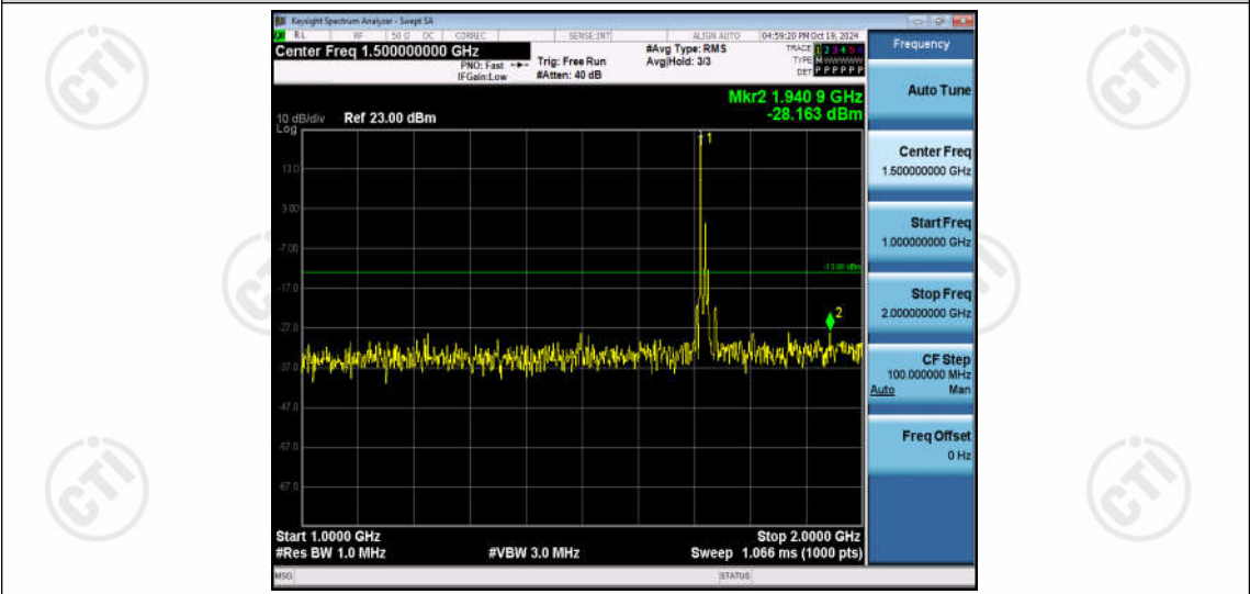
Band4-15MHz-QPSK-20025-1RB#0-Range2:1000~2000MHz
