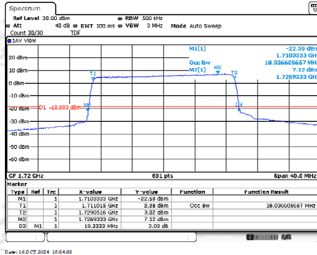
Band4-20MHz-QPSK-20050-100RB#0-18.037
