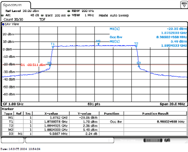
Band2-10MHz-QPSK-18900-50RB#0-8.985
