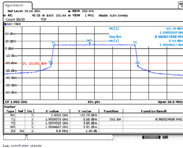
Band2-10MHz-QPSK-19150-50RB#0-8.985
