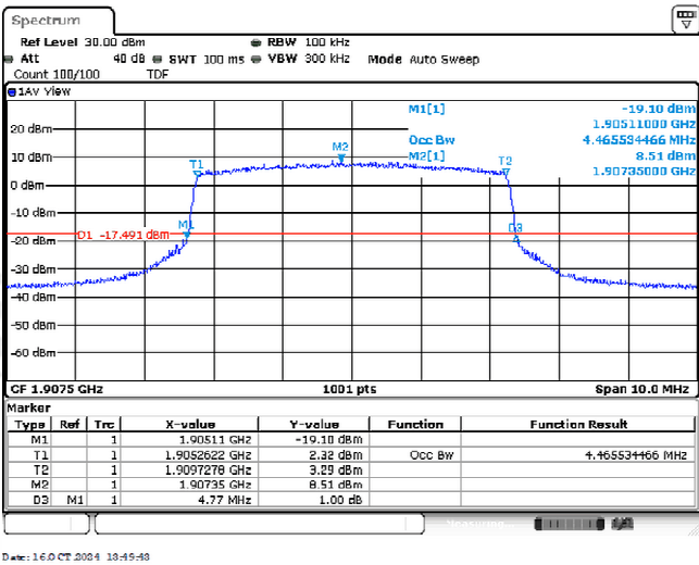
Band2-5MHz-QPSK-19175-25RB#0-4.466
