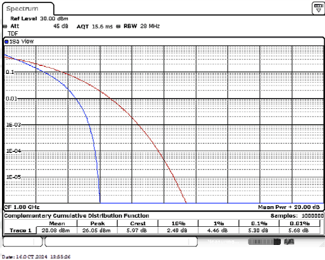
Band2-10MHz-QPSK-18900-50RB#0
