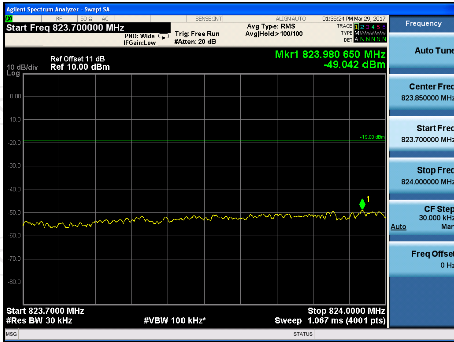
L-edge
