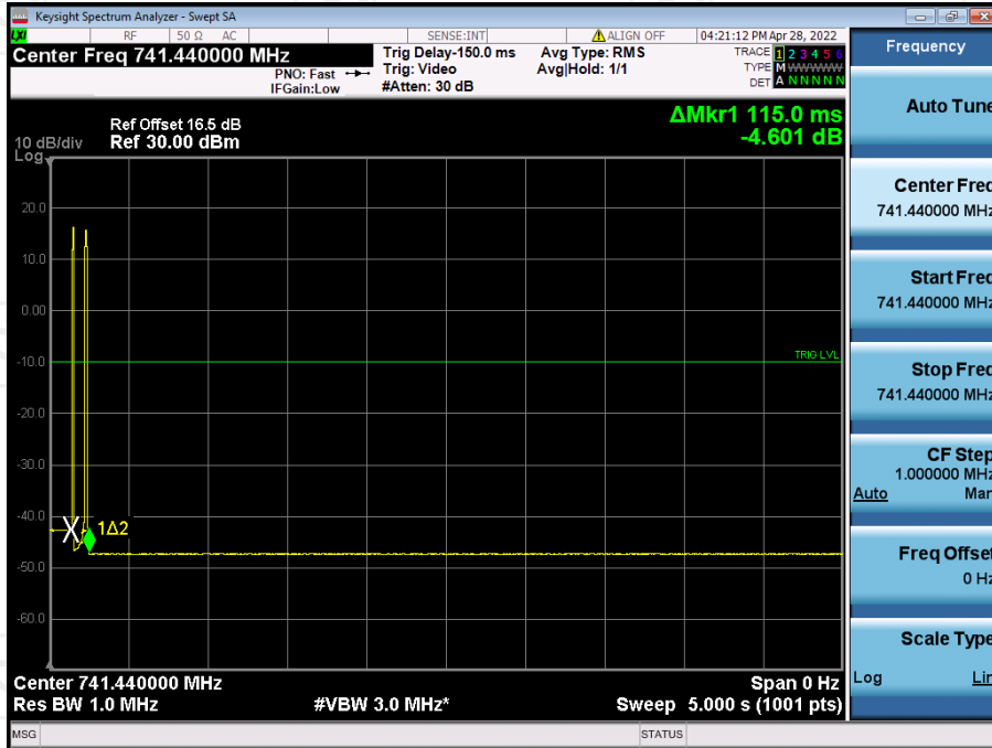
Lower700MHz DL
