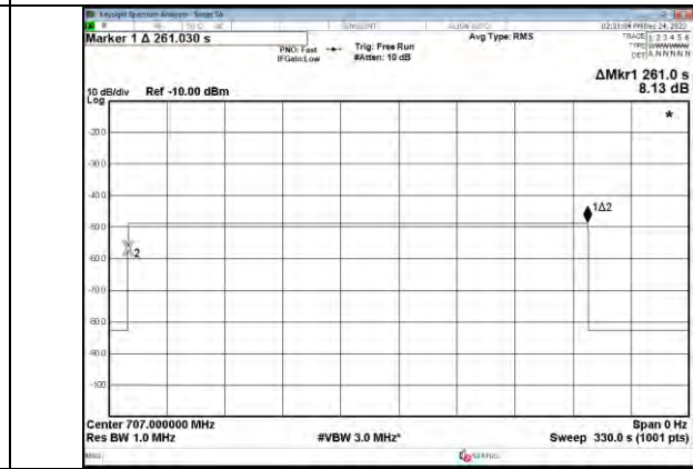
Lower 700MHz band
