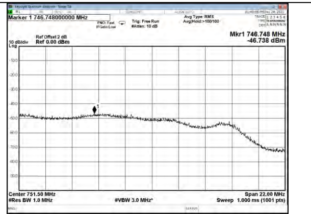
Upper 700MHz band DL
